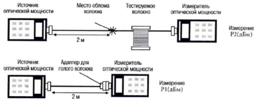
Рис. 1. Метод светопропускания: способ облома волокна
