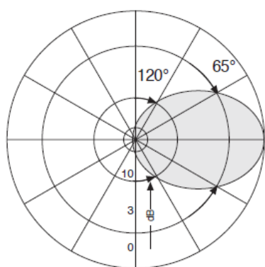
Рис. 2. Диаграмма направленности антенны k80010691
