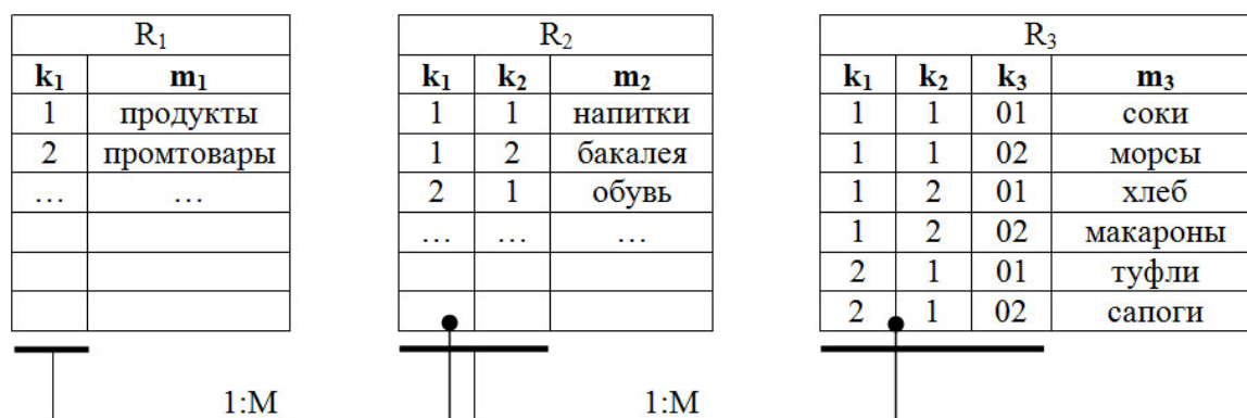
Рис. 2. 2NF нормализация отношения R^n|_{n=3}
