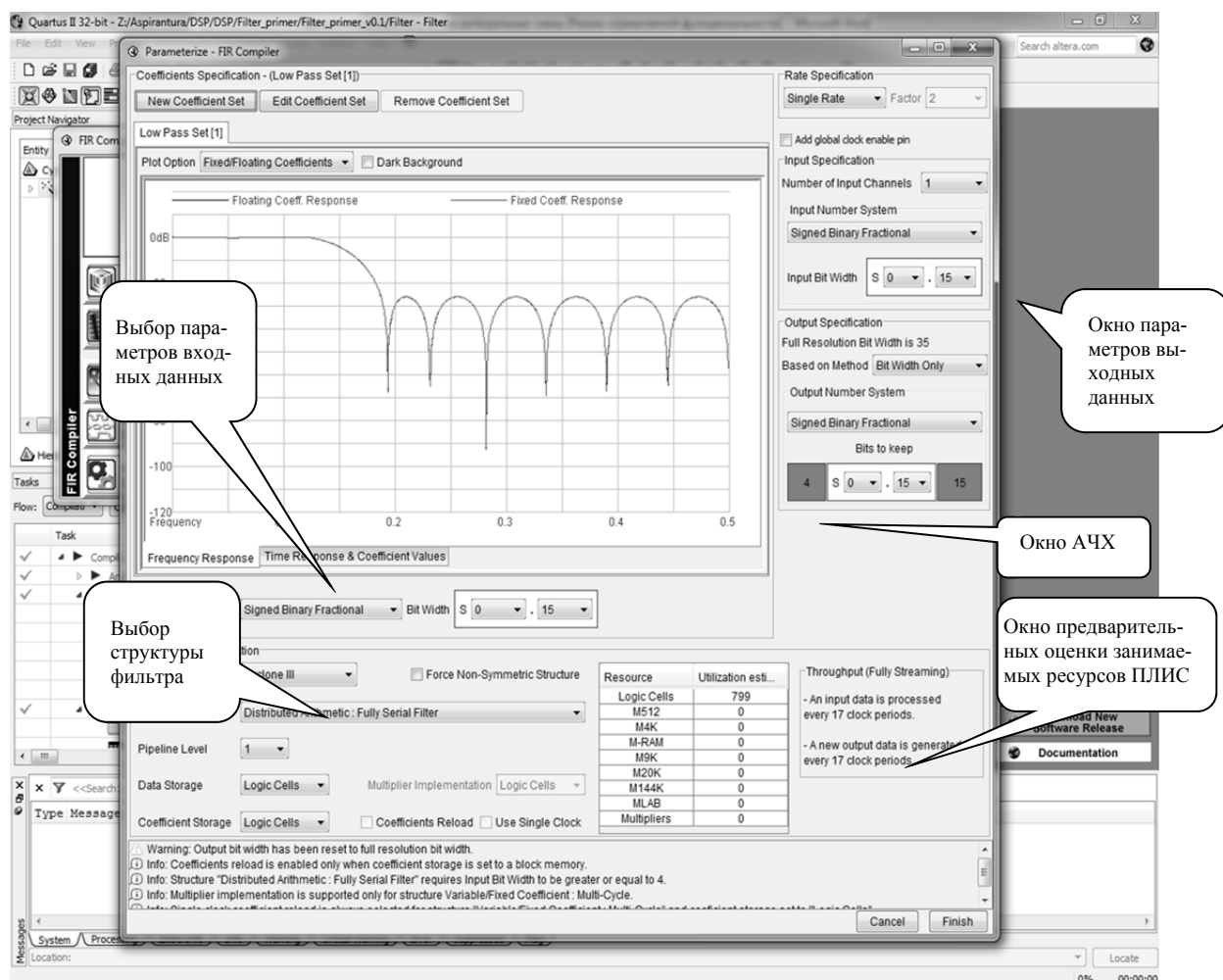
Рис. 1. Окно настроек и результата моделирования FIR Compiler
