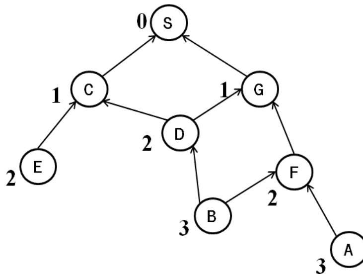
Рис. 3. Соединение в RPL
