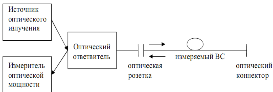
Рис. 2. Упрощенная схема измерения затухания ВС по методу обратного отражения
