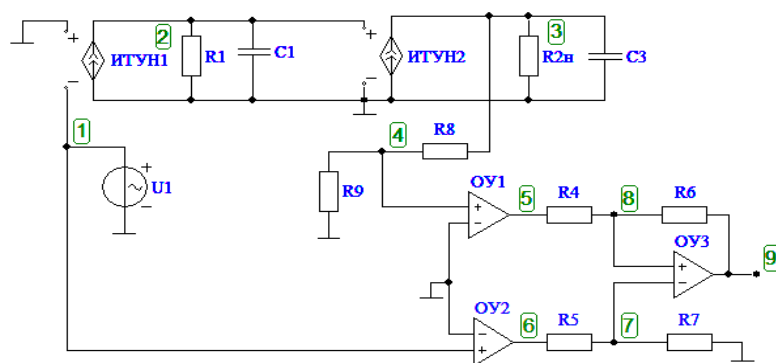
Рис. 2. Измерение глубины ОС
