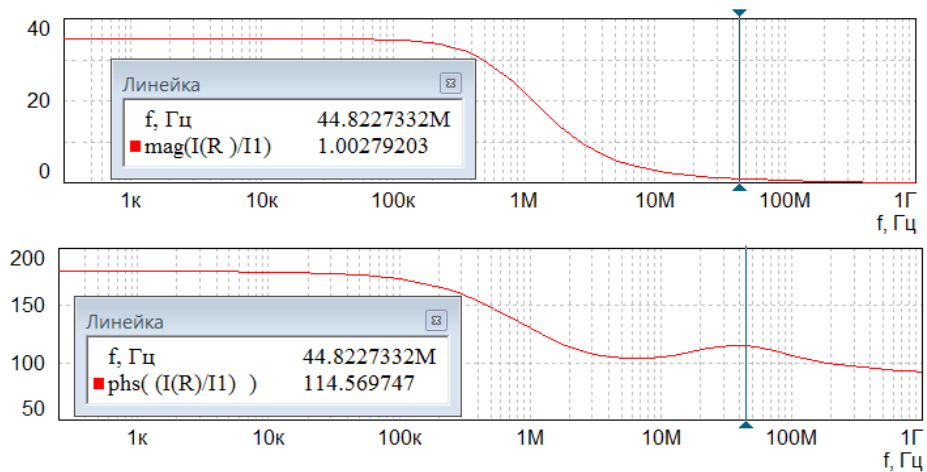
Рис. 8. АЧХ и ФЧХ петлевого усиления схемы рис. 7
