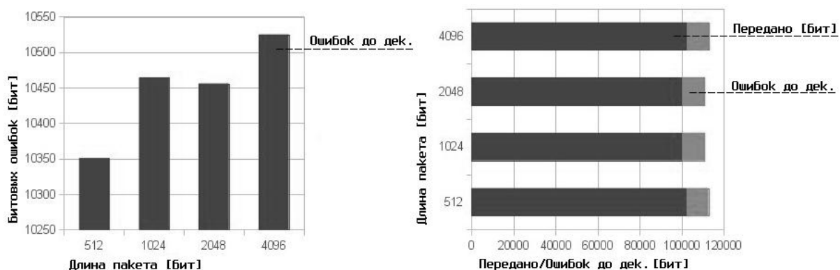
Рис. 1. Диаграммы передачи данных при соотношении E_b/N_0=0.79
