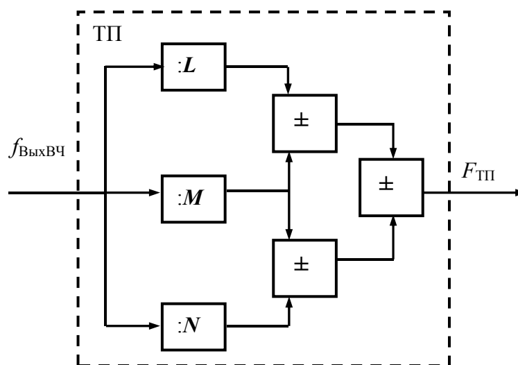
Рис. 3. Структура двойного целочисленного нониусного ТП
