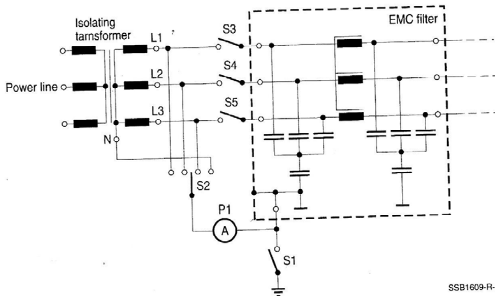
Рис. 5. Измерение тока утечки в трехфазных трехпроводных IT-цепях (Epcos)
