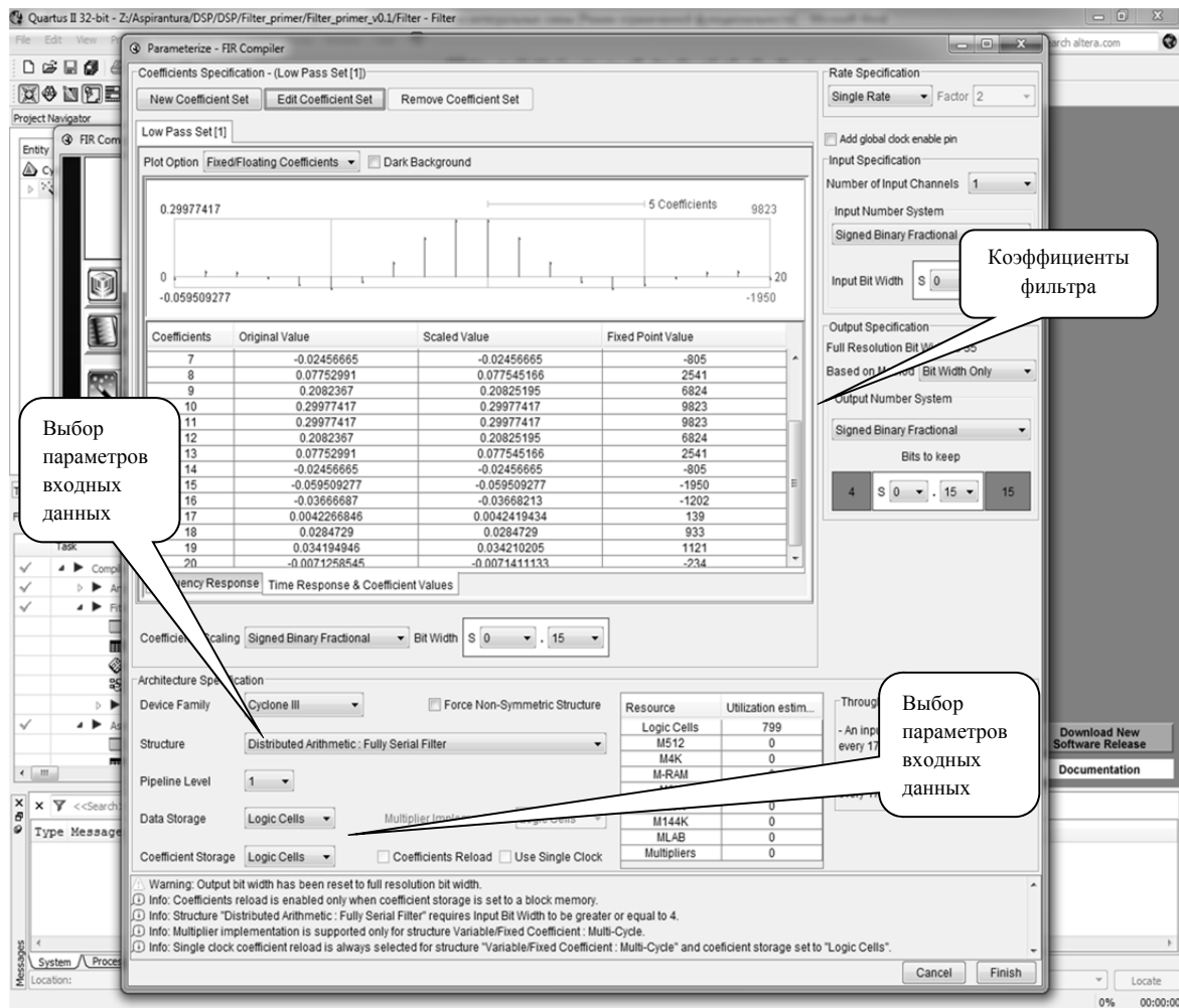
Рис. 2. Окно настроек и моделирования FIR Compiler
