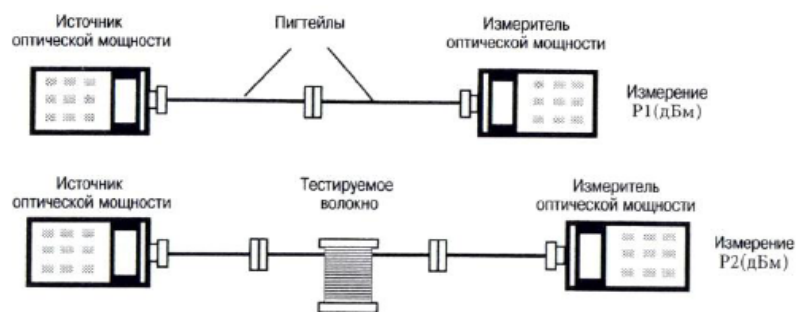
Рис. 2. Метод светопропускания: способ вносимых потерь
