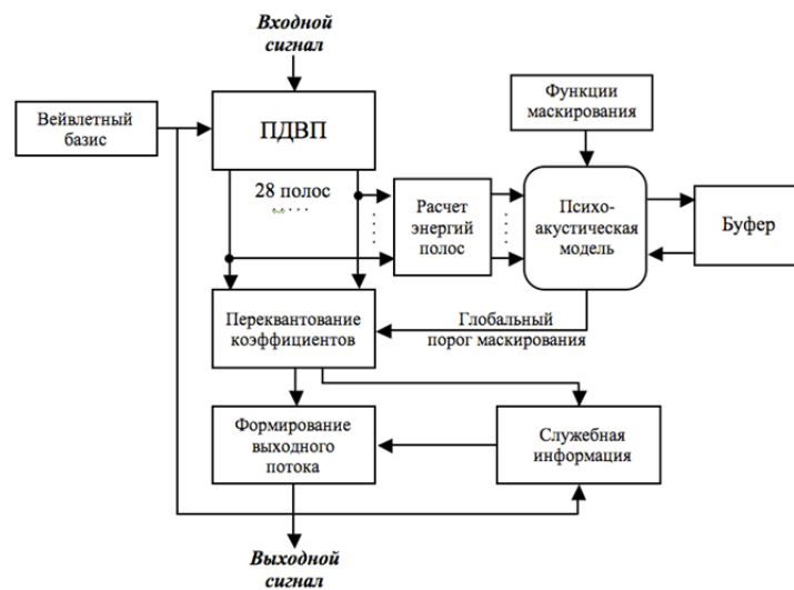
Рис. 1. Структурная схема экспериментального вейвлетного кодера [1]
