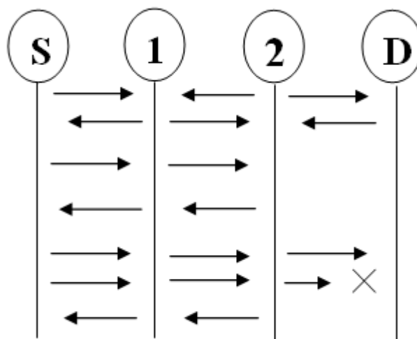
Рис. 2. Обмен сообщениями в протоколе AODV
