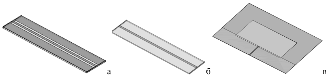
Рис. 1. Модель копланарного волновода (а), модель микрополосковой линии (б), модель антенной системы с копланарным волноводом (в)
