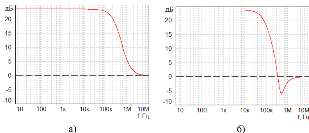
Рис. 3. АЧХ глубины ОС однополюсной а) и двухполюсной б) функции передачи.
