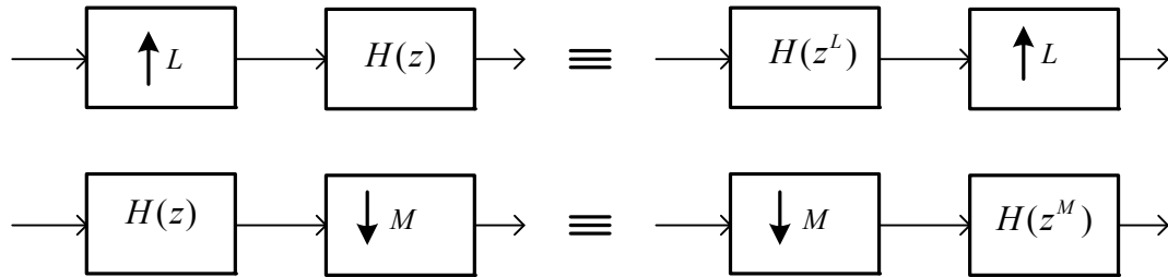
Рис. 1. Замечательные тождества для систем однократной интерполяции (верхнее) и децимации (нижнее)
