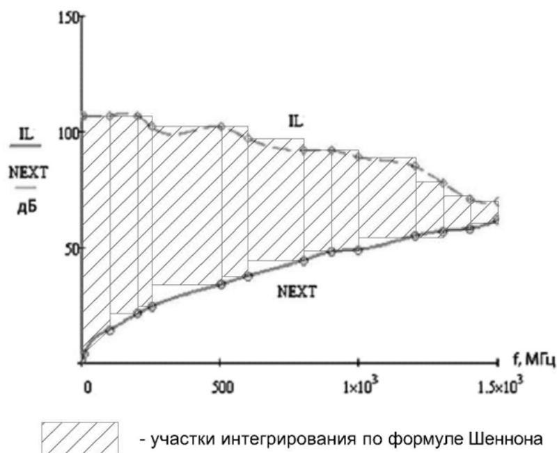
Рис. 2. Графики вносимого затухания (IL) и переходного затухания на ближнем конце (PS-NEXT)
