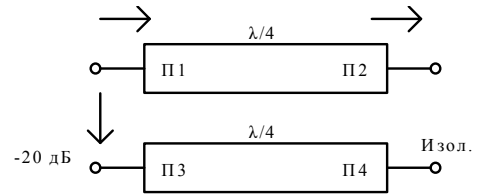
Рис. 1. Идеальный НО с обратной связью, реализованный на четвертьволновых отрезках линии и переходным затуханием C = 20 дБ
