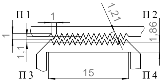
Рис. 5. Топология зубчатого НО
