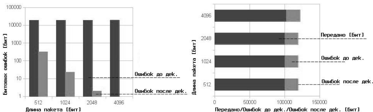
Рис. 2. Диаграммы передачи данных при соотношении E_b/N_0=0.39
