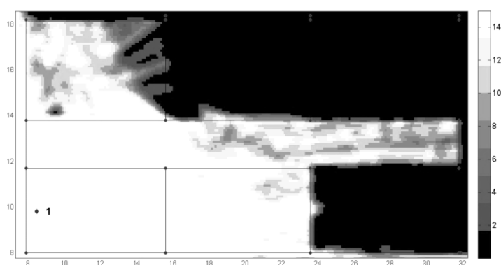
Рис. 2. Распределение CQI для первой фемтосоты
