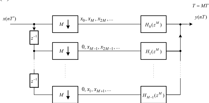
Рис. 3. Полифазная структура системы однократной децимации
