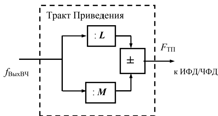
Рис. 2. Структура одинарного целочисленного нониусного ТП
