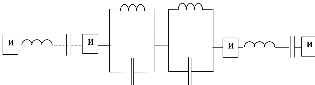
Рис. 2. Схема эллиптического полосового фильтра – прототипа 3 порядка, после введения инверторов
