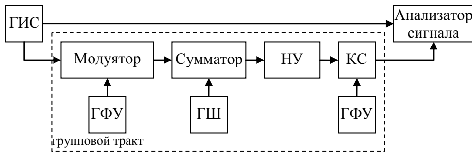
Рис. 1. Функциональная схема модели группового тракта:
