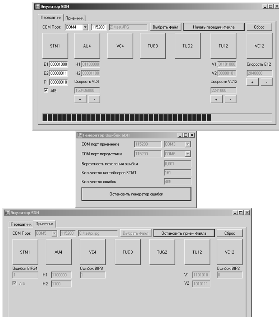
Рис. 4. Процесс передачи файла с внесением ошибок. Процесс пойман в момент цифровой коррекции по прямой линии в TU-12
