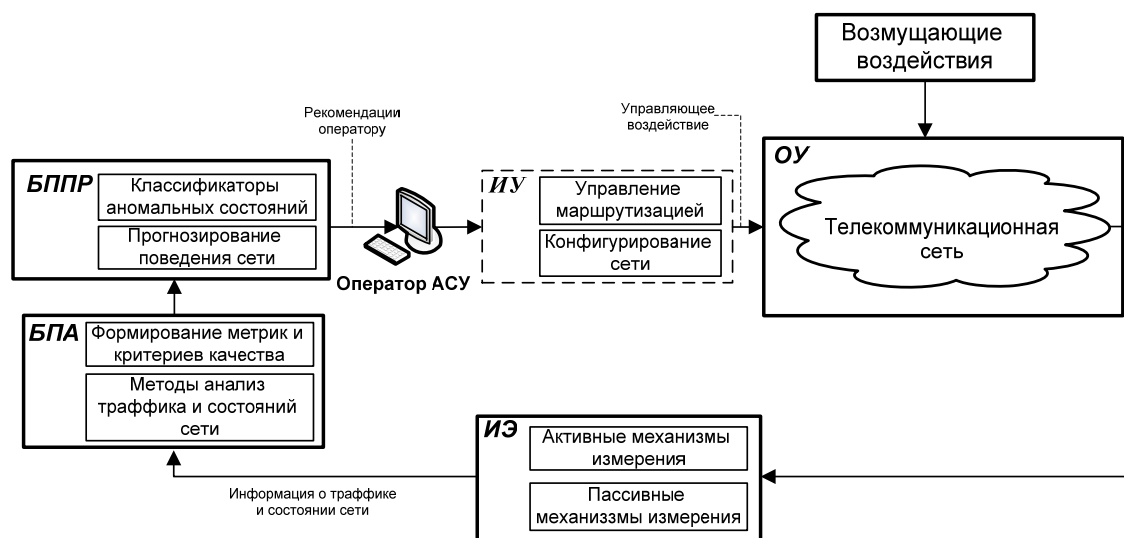
Рисунок. Модель АСУ телекоммуникационной сетью
