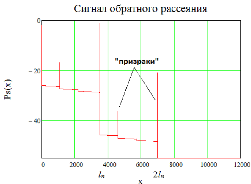
Рис. 2. Сигнал обратного рассеяния
