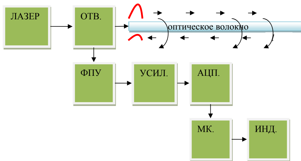
Рис. 1. Структурная схема оптического рефлектометра
