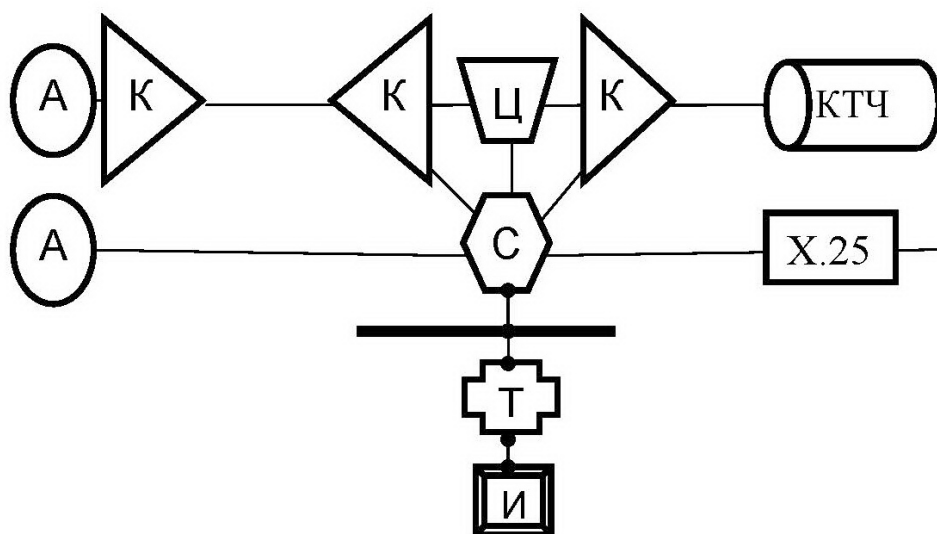
Рис. 1. Структурная схема Санкт-Петербургского узла телеграфной связи:
