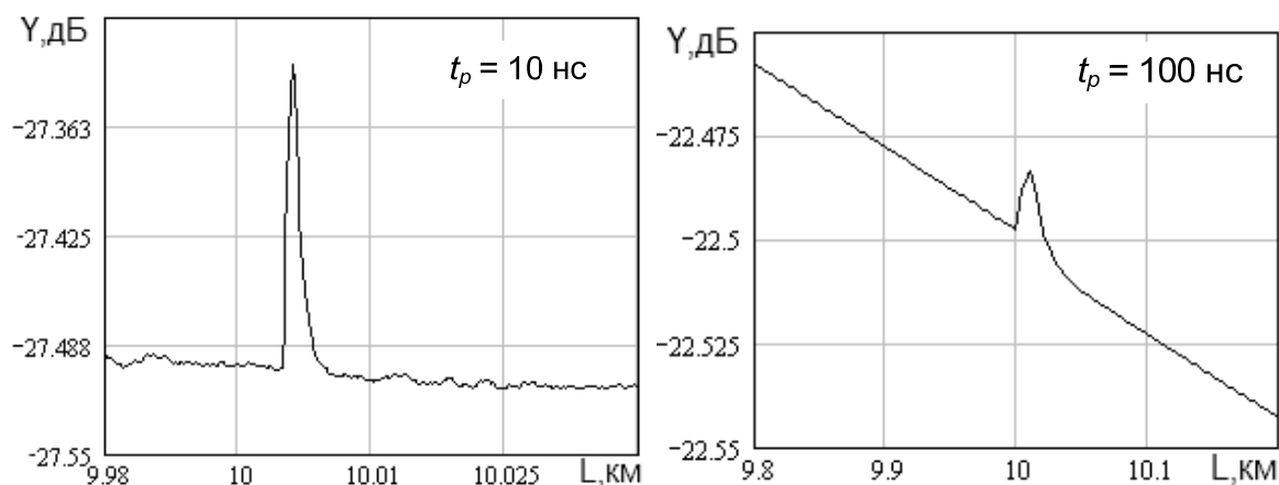
Рис. 2. Результаты моделирования COP при l_n = 10 км
