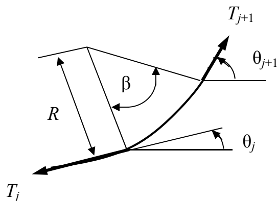
Рис. 3. Вертикальный изгиб кабеля при прокладке
