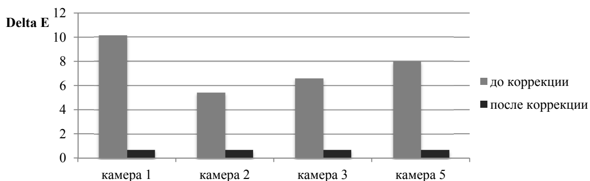
Рис. 3. Значения средней величины цветового различия изображений, полученных с камер многокамерной системы, до и после коррекции
