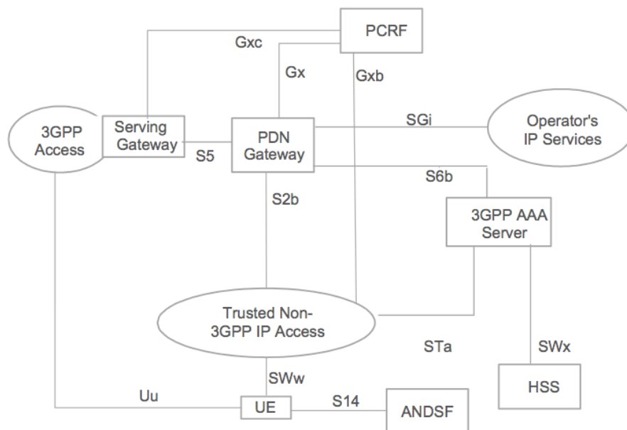
Рис. 3. Архитектура ядра сети LTE с доверенным доступом
