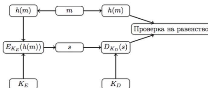
Рис. 3. Схема аутентификации исполняемого кода
