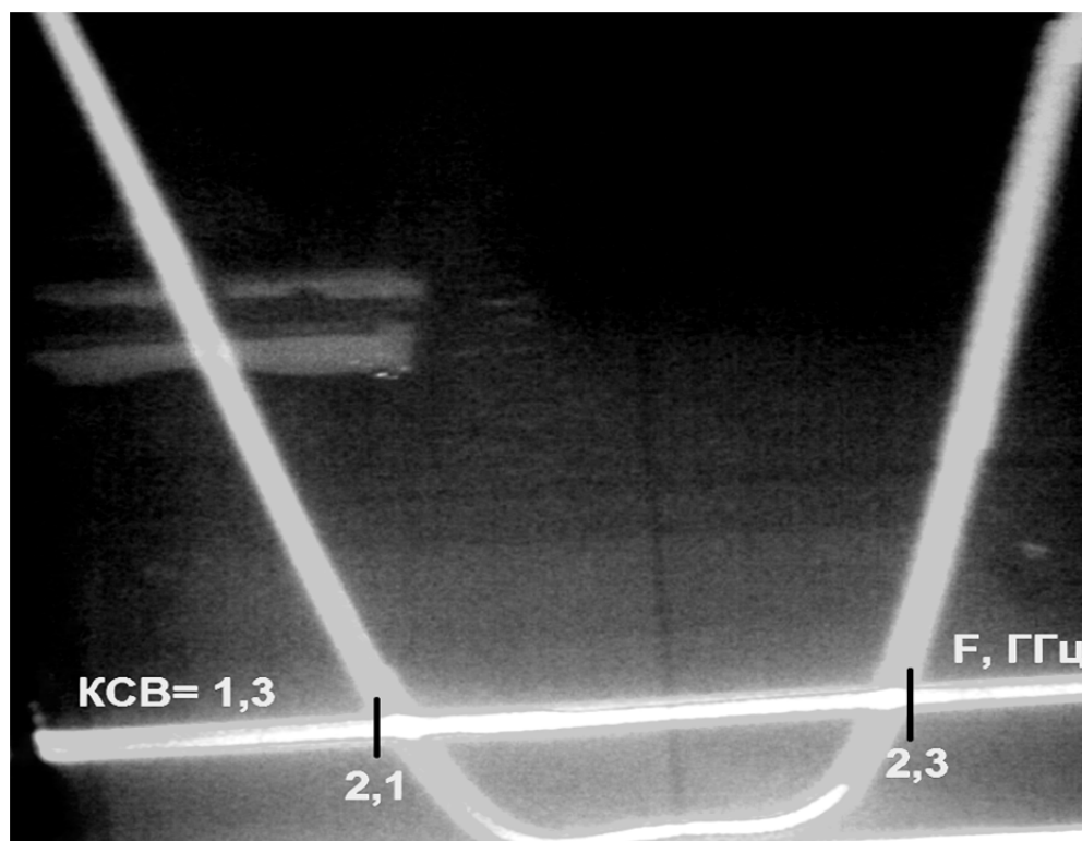
Рис. 2. КСВ антенны согласованной устройством на компланарном волноводе
