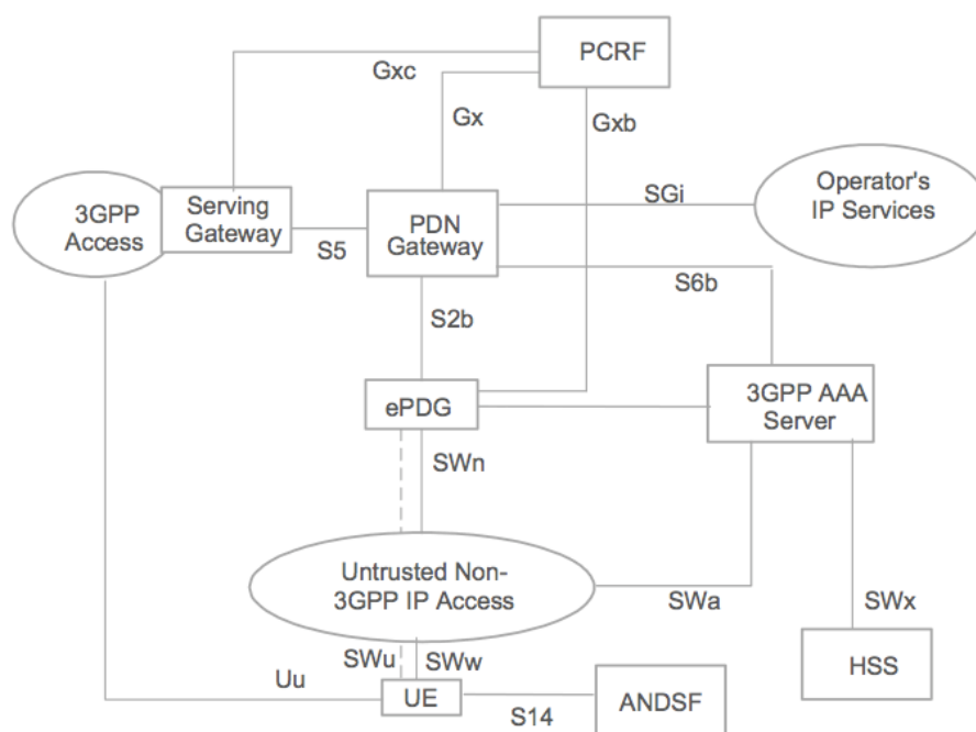
Рис. 2. Архитектура ядра сети LTE с недоверенным доступом
