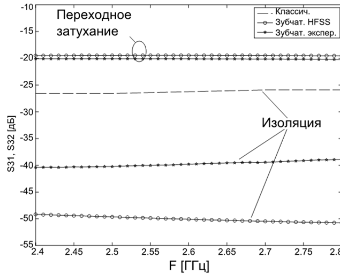
Рис. 4. Экспериментальные и теоретические переходное ослабление S_{31} и изоляция S_{32} классического микрополоскового НО и зубчатого
