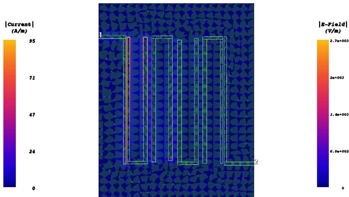
Рис. 4. Распределения плотности токов на поверхности металлического проводника и электрического поля внутри и вне диэлектрика шпилечного фильтра 2D
