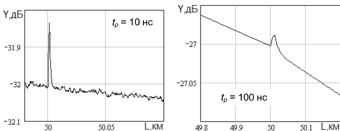
Рис. 3. Результаты моделирования COP при l_n = 50 км.
