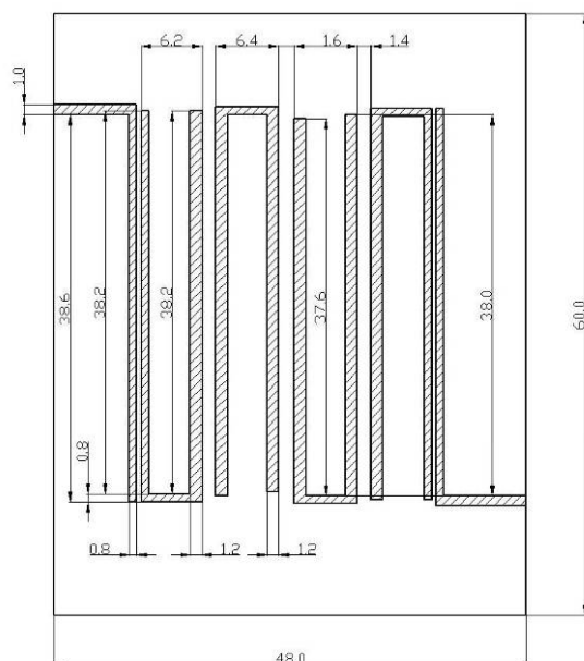
Рис. 3. Топология шпилечного фильтра четвертого порядка с геометрическими размерами
