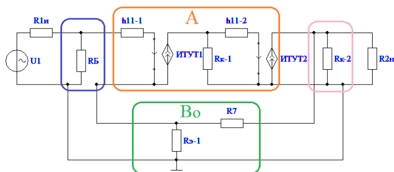
Рис. 2. Структура ОС в схеме Блэка
