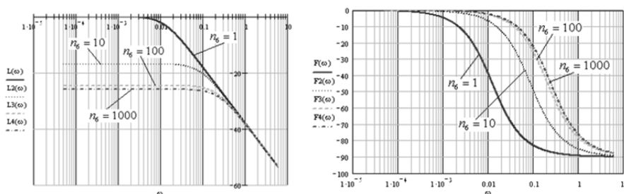
Рис. 5. Логарифмические амплитудно-частотные характеристики и фазо-частотные характеристики при n_6=1 , n_6=10 , n_6=100 , n_6=1000
