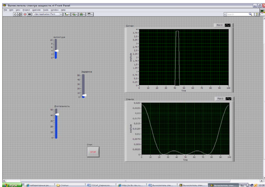
Рис. 3. Лицевая панель виртуального прибора
