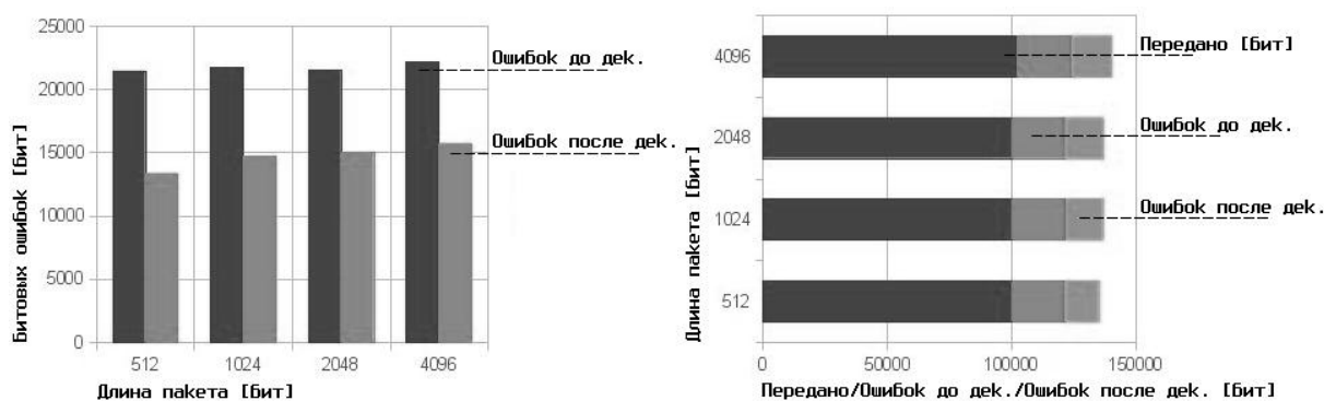
Рис. 3. Диаграммы передачи данных при соотношении E_b/N_0=0.25
