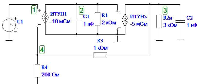
Рис. 1. Эквивалентная схема усилителя с ОС
