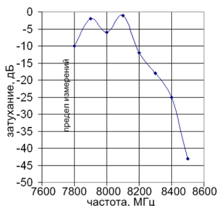
Рис. 3. Экспериментальная характеристика затухания лабораторного макета гребенчатого фильтра 5-го порядка с цилиндрическими резонаторами до оптимизации
