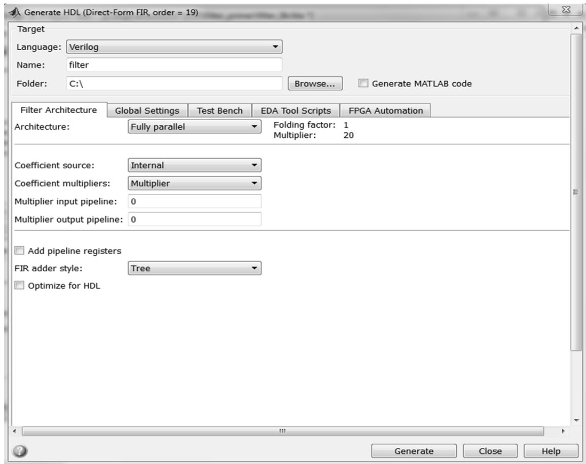
Рис. 2. Окно Generate HDL
