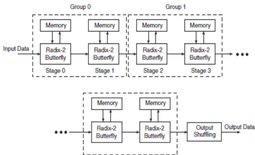
Рис. 1. Поточковый конвейерный алгоритм БПФ
