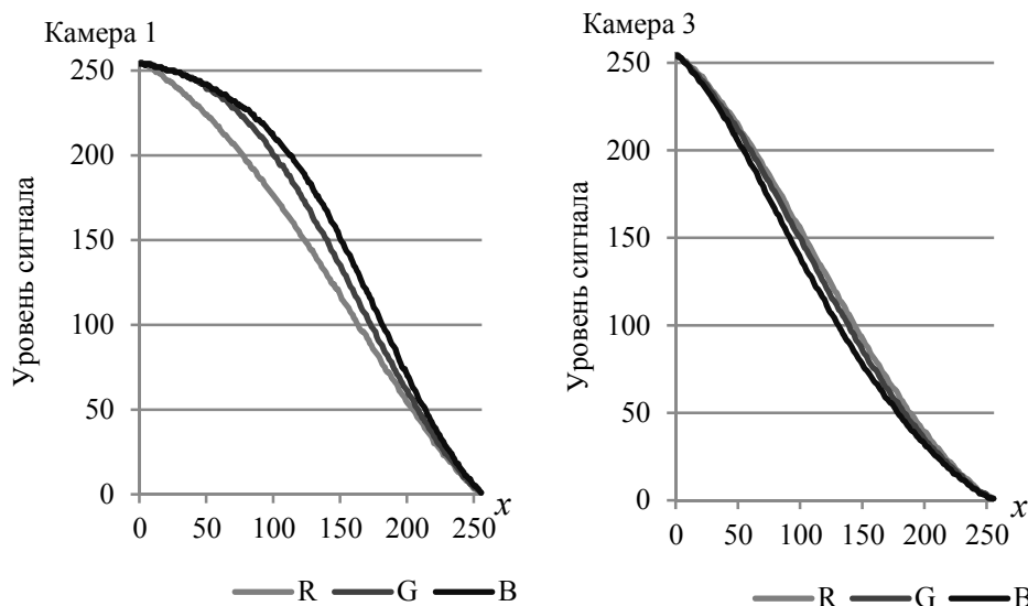
Рис. 2. Характеристики цветовой чувствительности двух камер многоракурсной системы для R , G и B каналов
