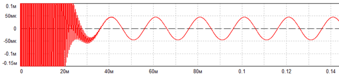
Рис. 4. График тока утечки через эквивалент человека
