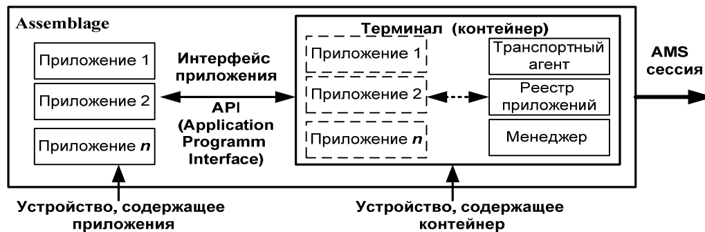
Рис. 4. AMS сборка
