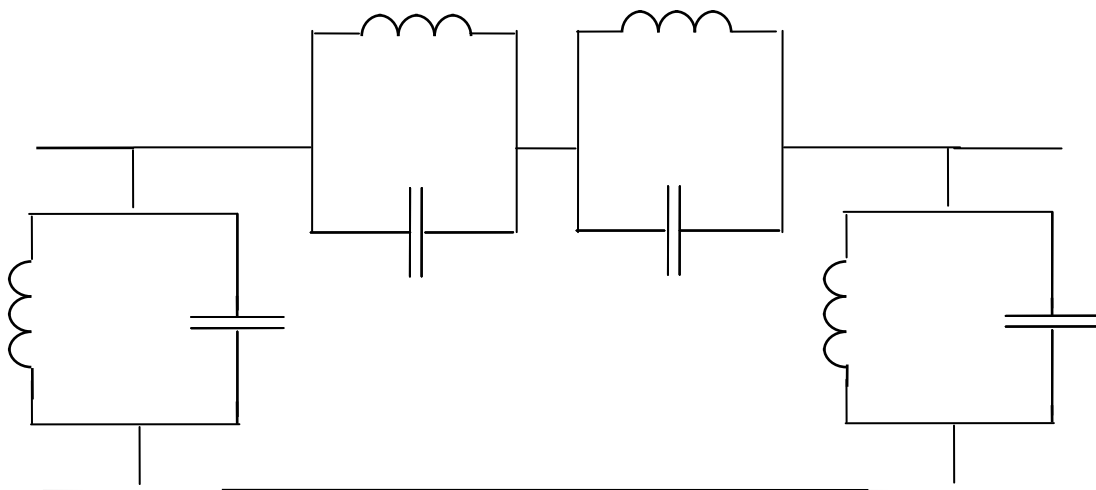
Рис. 1. Схема эллиптического полосового фильтра – прототипа 3 порядка
