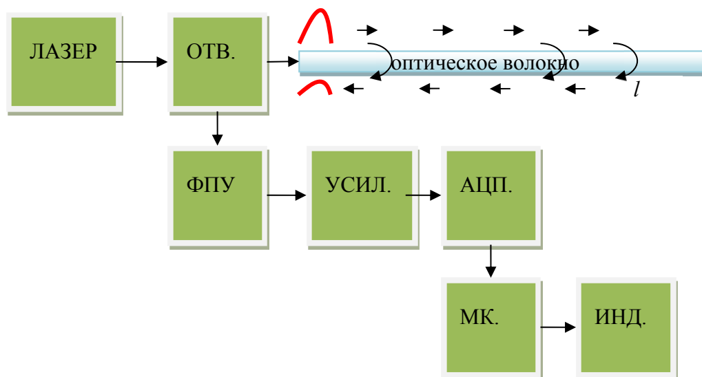
Рис. 1. Структурная схема рефлектометра построенного по классической схеме
