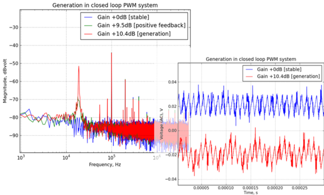
Рис. 4. Увеличение усиления по петле ООС до момента возникновения генерации (проверка запасов устойчивости)
