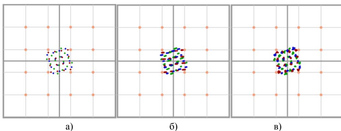
Рис. 2. Графики КАМ созвездий на 3-х поднесущих символа OFDM: а) с добавлением ЦП; б) без ЦП; в) без ЦП с добавлением аддитивного шума в канале.
