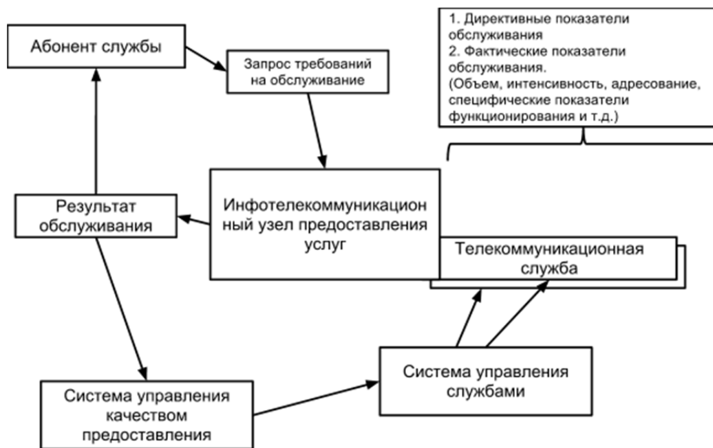
Рис. 5. Современный узел предоставления услуг
