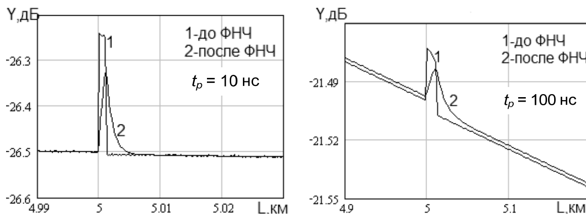
Рис. 1. Результаты моделирования СОР при l_n = 5 км
