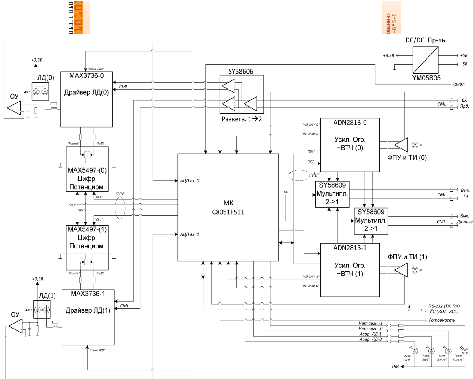
Рис. 1. Функциональная схема ОУТ
