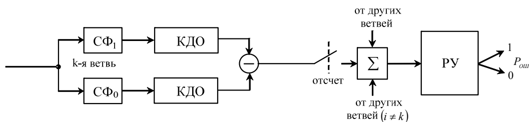
Рис. 1. Схема НК квадратичного сложения сигналов при n ветвях разнесения по времени прихода лучей
