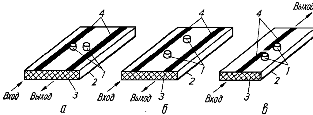
Рисунок. Полосно-пропускающие фильтры на основе микрополосковых линий с ДР
