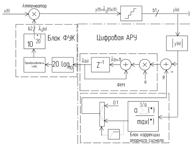
Рис. 4. Структурная схема модели ЦАРУ с блоком коррекции опорного сигнала
