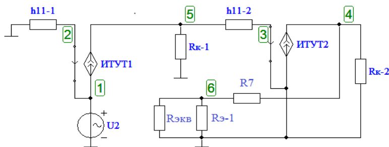
Рис. 3. Разрыв петли ОС в пассивной части цепи
