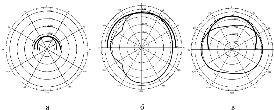
Рис. 3. Диаграмма направленности микрополосковой линии (а), прямоугольного излучателя (б), антенной системы с микрополосковой линией (в)
