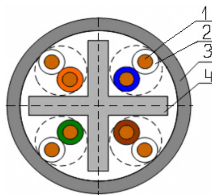
Рисунок. Поперечное сечение кабеля: 1 – медные токоведущие жилы; 2 – изоляция жил; 3 – оболочка кабеля; 4 – сепаратор
