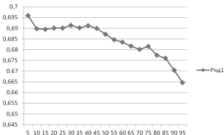
Рис. 2. Зависимость показателя Хёрста от уровня потерь
