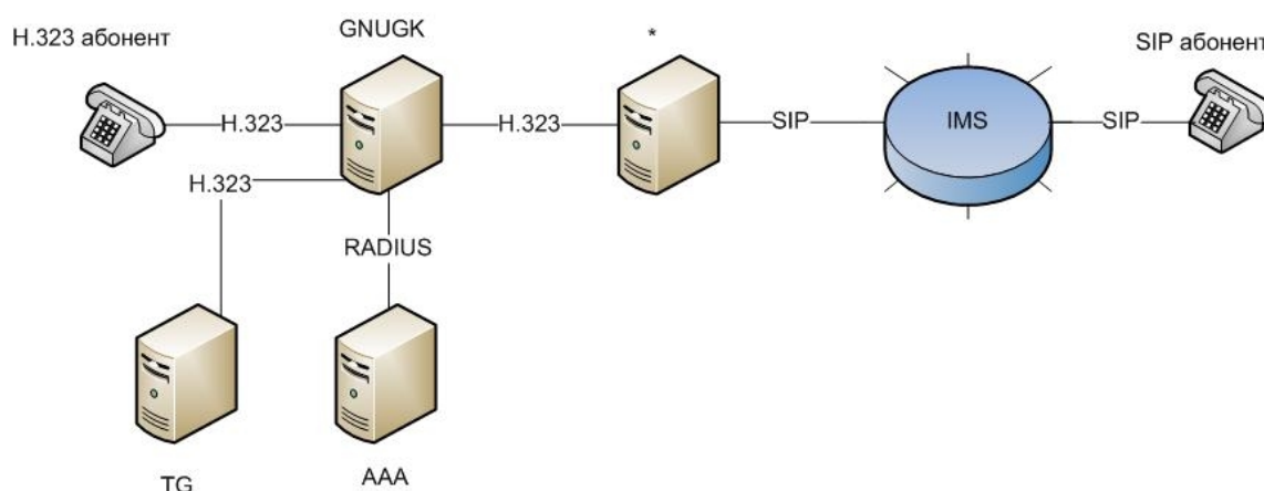
Рис. 1. Архитектура сети, на которой проводилось физическое моделирование
