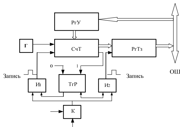
Рис. 1. Блок-схема устройства
