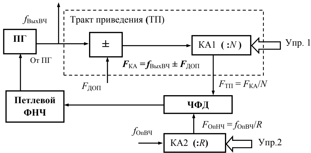
Рис. 1. Обобщенная структура кольца импульсно-фазовой автоподстройки частоты (ИФАП)
