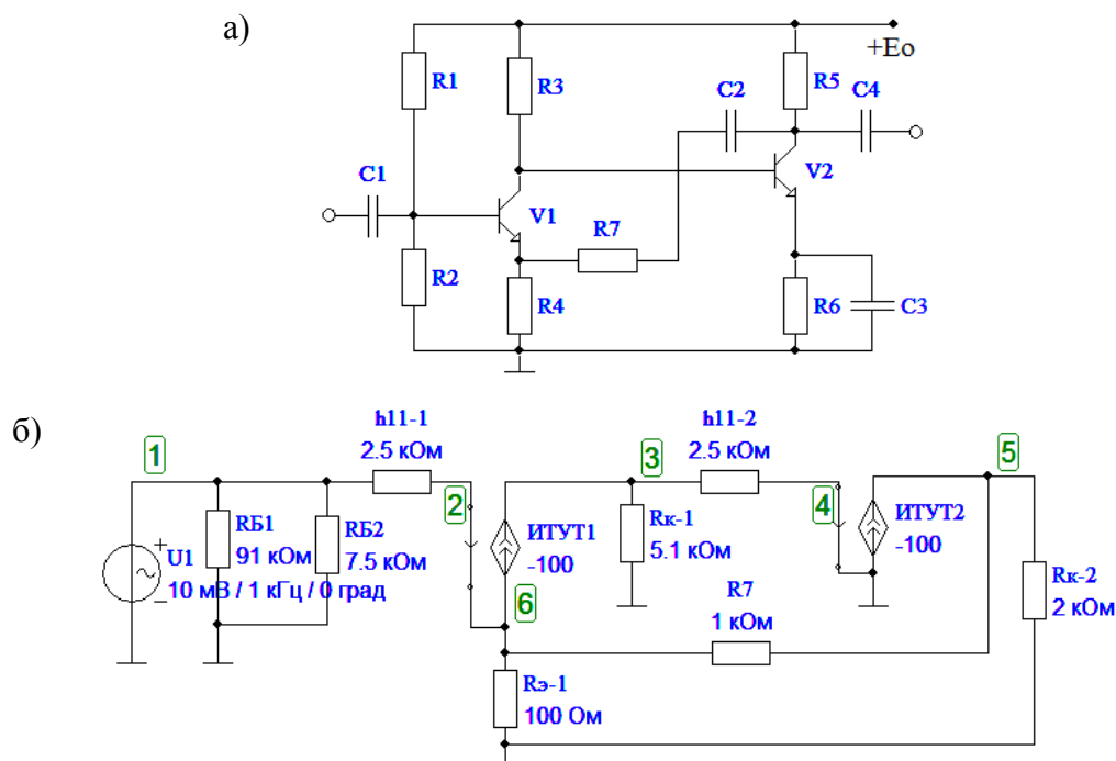
Рис. 1. Схема Блэка а) и её эквивалентная схема для средних частот б)
