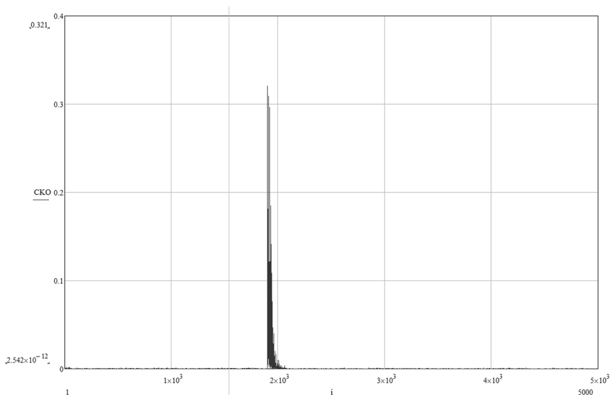
Рисунок. График зависимости СКО от номера итерации при дисперсии шума 10^{-4} . На 1900 итерации импульсная характеристика была изменена. Можно увидеть, что скорость сходимости алгоритма весьма высока
