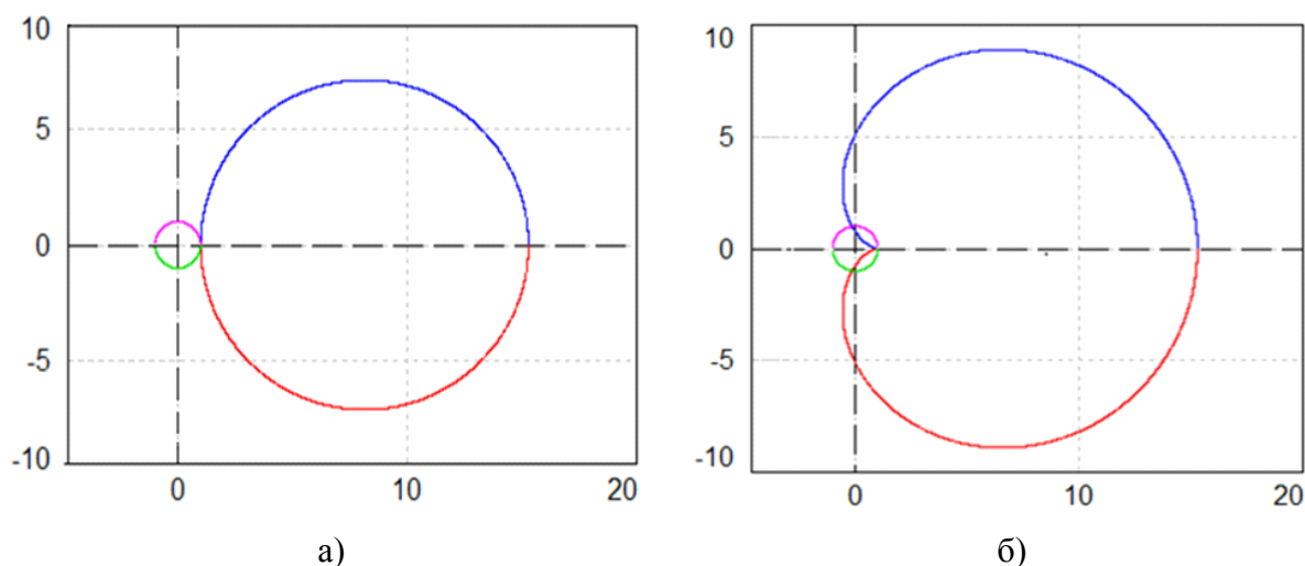
Рис. 4. Годограф возвратной разности при однополюсной а) и двухполюсной б) функции передачи
