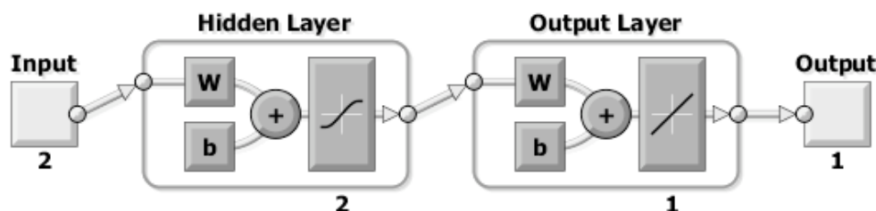
Рисунок. Вид созданной нейронной сети в системе MATLAB
