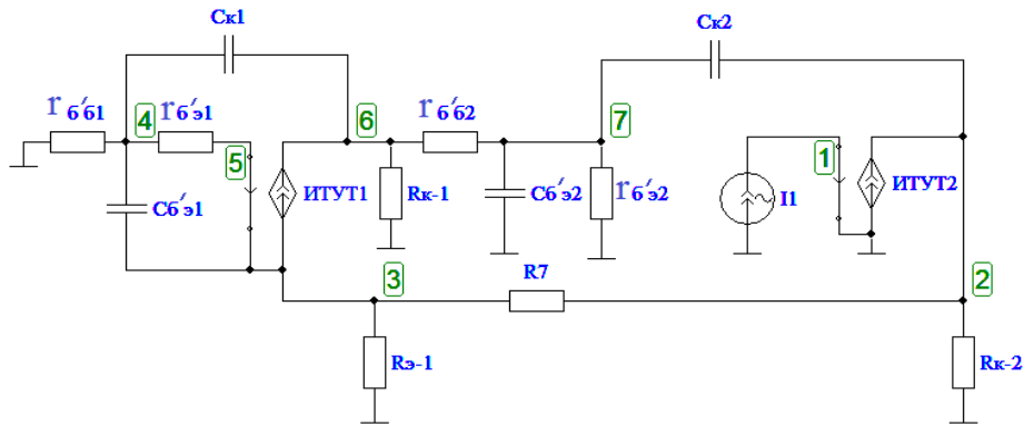
Рис. 7. Эквивалентная схема разомкнутой петли ОС для области ВЧ
