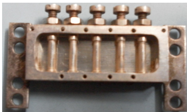
Рис. 1. Лабораторный макет гребенчатого фильтра 5-го порядка с цилиндрическими резонаторами
