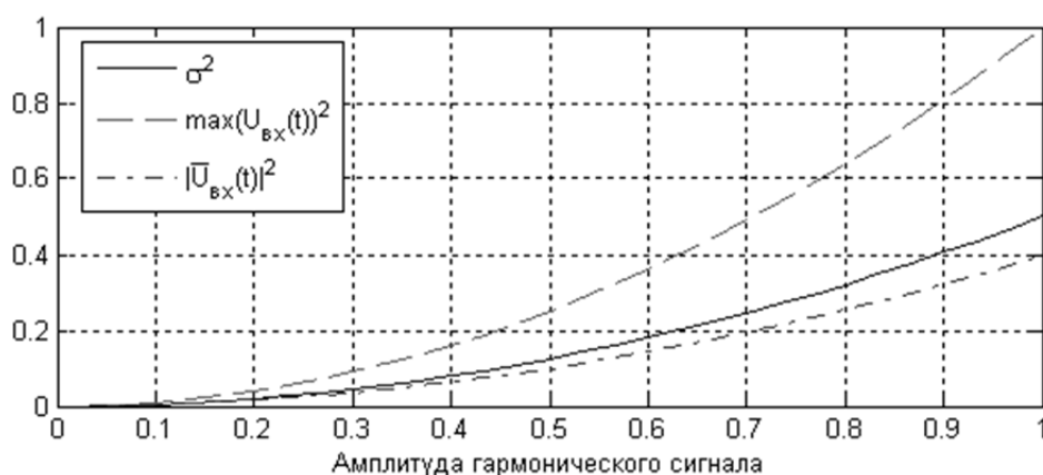
Рис. 2. Энергетические характеристики сигнала (дисперсия, квадрат максимального значения, квадрат среднего значения огибающей)
