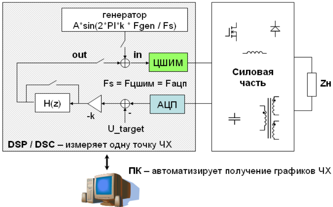
Рис. 3. Встроенный цифровой измеритель ЧХ петлевого усиления
