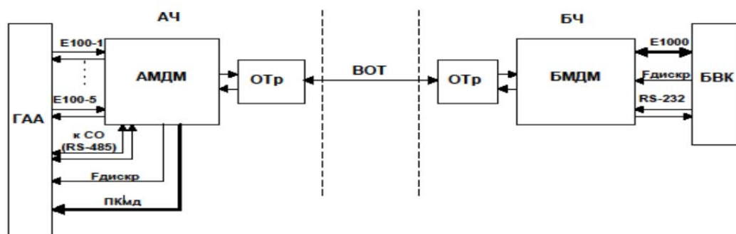
Рисунок. Структурная схема ВОСПИ
