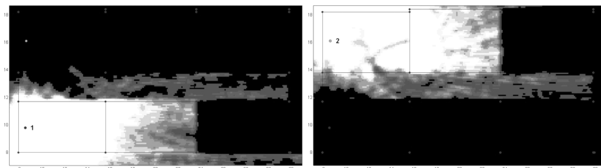
Рис. 6. Распределение CQI для фемтосот 1 и 2 (сценарий 4)
