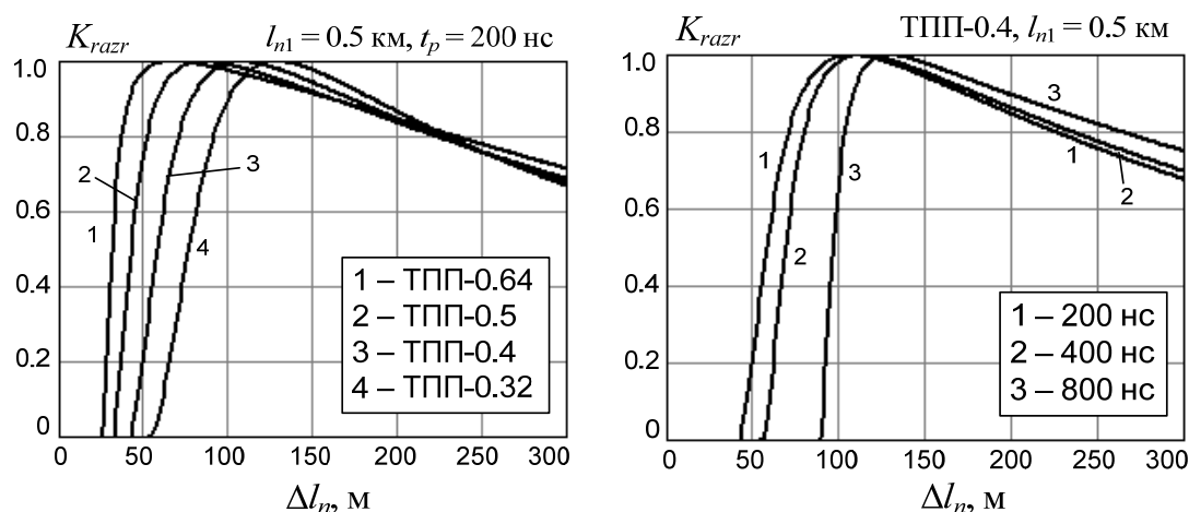
Рис. 2. Зависимости коэффициента разрешения от \Delta l_n для различных кабельных цепей (слева) и длительностях ЗИ (справа)
