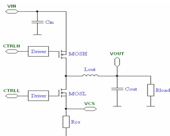
Рис. 1. Типовая схема силовой части усилителя с ШИМ
