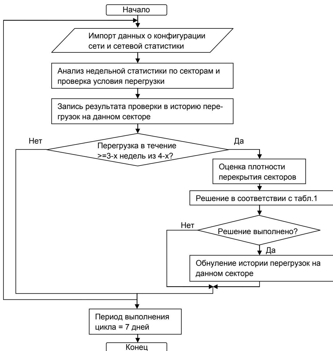
Рис. 2. Алгоритм принятия решения об активации дополнительных несущих
