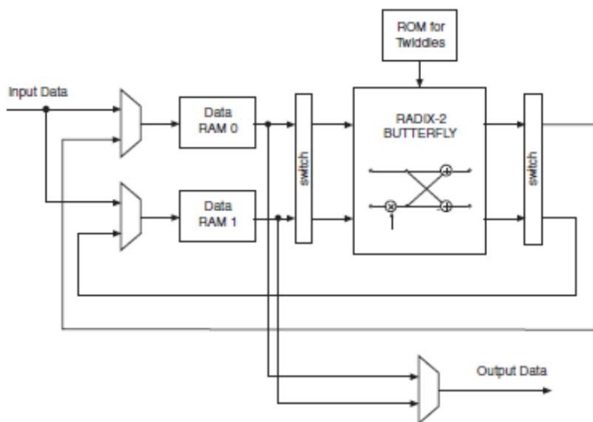
Рис. 2. Пакетный алгоритм БПФ «бабочкой» основанию 2
