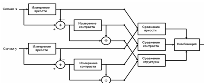
Рис. 2. Схема вычисления метрики SSIM
