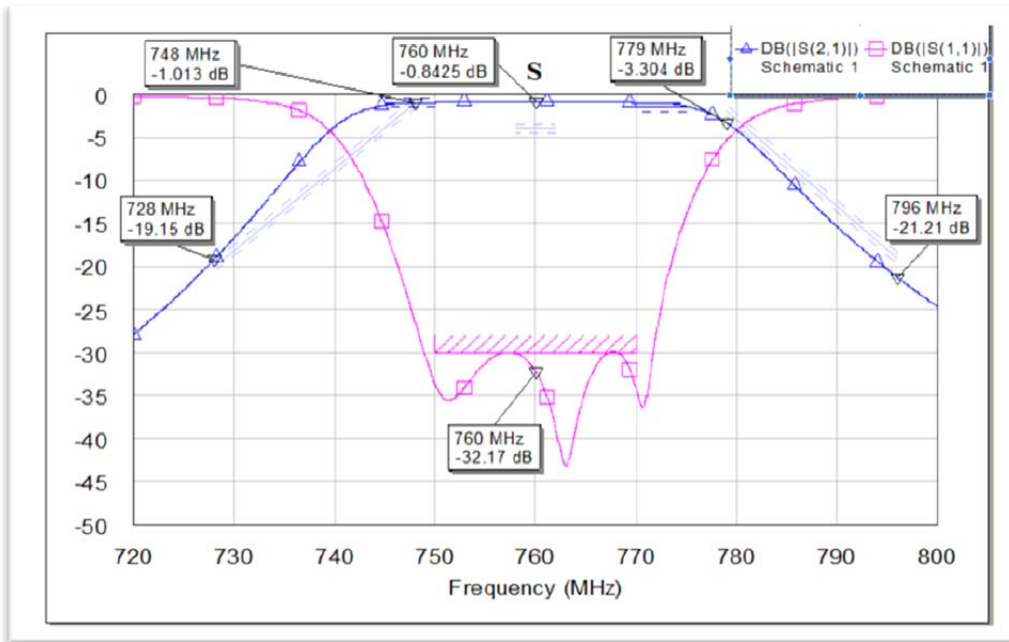
Рис. 5. Характеристики затухания (S21) и коэффициента отражения на входе (S11) фильтра
