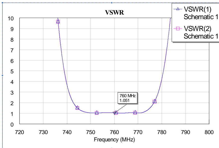
Рис. 6. Характеристики КСВН вх/вых фильтра
