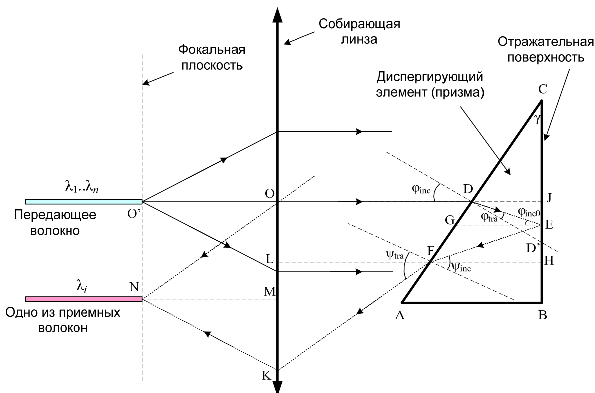
Рисунок. Демультиплексор на отражательной призме, построенный по схеме Литтроу
