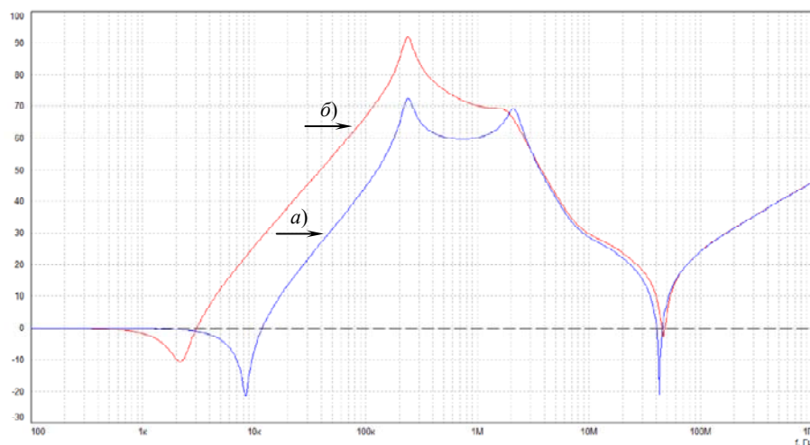
Рис. 11. График подавления ФРП для несимметричных помех: а) без компенсации; б) с активной компенсацией
