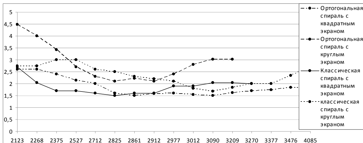
Рис. 5. Зависимости КСВН ОС от вида экрана
