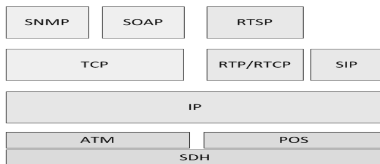
Рис. 2. Типовой стек протоколов внутриобъектовой сети связи
