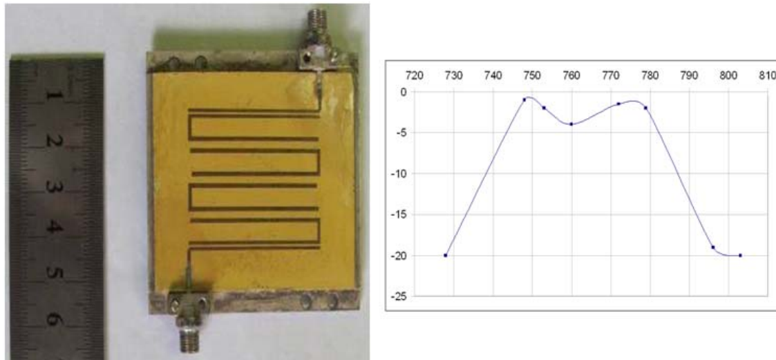
Рис. 1. Экспериментальный макет шпилечного фильтра и экспериментальная зависимость затухания лабораторного макета шпилечного фильтра четвертого порядка от частоты
