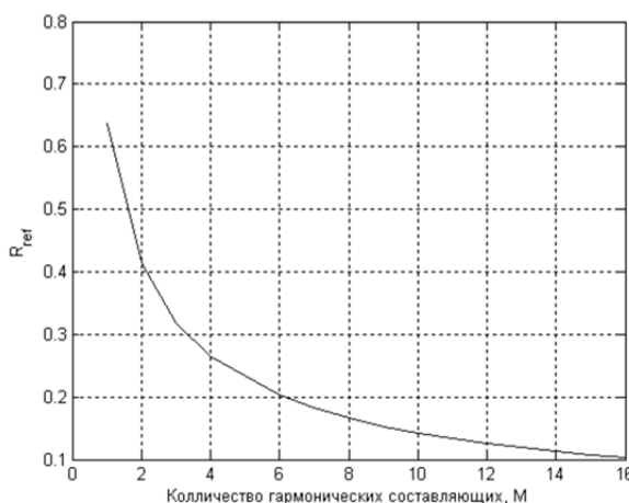
Рис. 3. Зависимость \frac{|\bar{U}_{вх}(t)|}{\max(U_{вх}(t))} относительно числа гармонических составляющих ( M )
