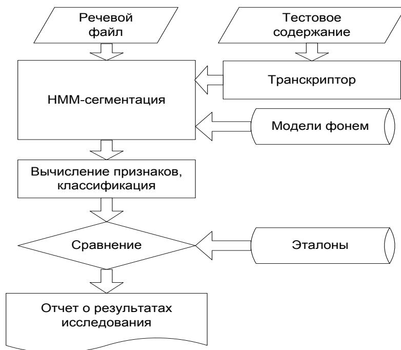
Рисунок. Функциональная схема АПК
