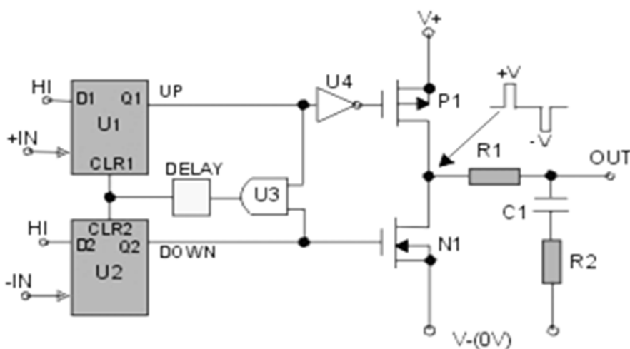
Рис. 2. Реализация ЧФД на D-триггерах и схемы подкачки заряда на комплементарной паре полевых транзисторов
