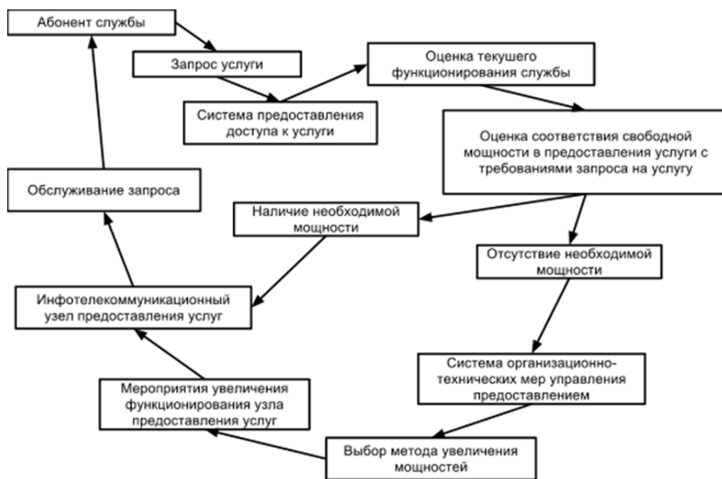
Рис. 4. Алгоритм включения службы в инфотелекоммуникационный узел
