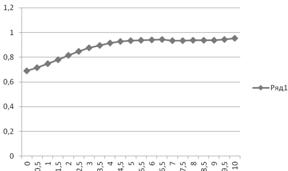
Рис. 3. Зависимость показателя Хёрста от скорости суммарного входного потока, Мбит/с
