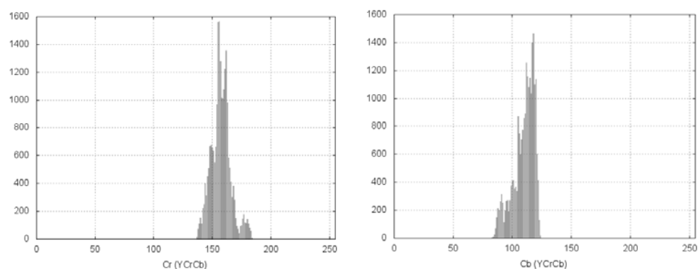
Рис. 4. Распределение цвета кожи из тестового набора в YCrCb -пространстве.
