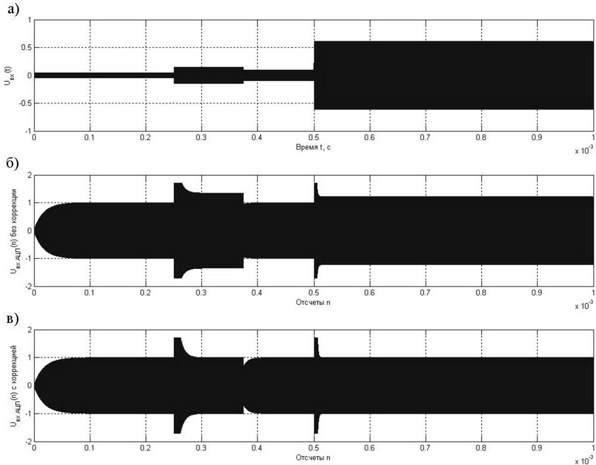
Рис. 5. Результат моделирования работы системы ЦАРУ при подаче: а) входного сигнала; б) без блока коррекции опорного сигнала; в) с блоком коррекции опорного сигнала
