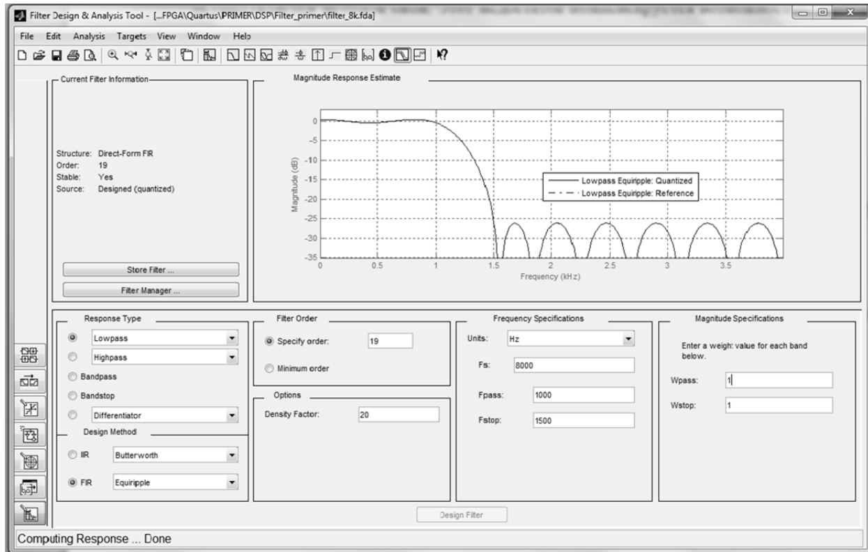
Рис. 1. Результаты моделирования фильтра в среде FDATool с заданными параметрами
