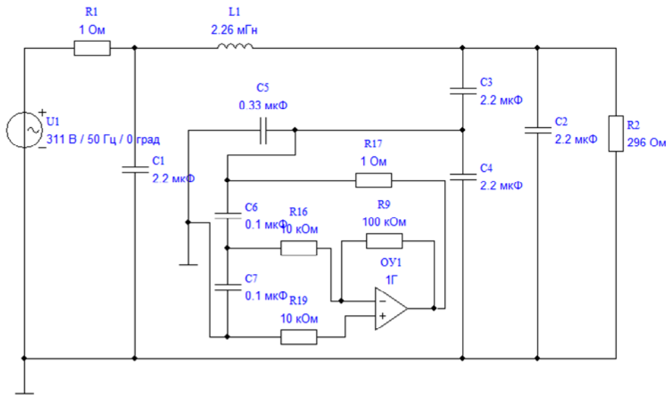
Рис. 9. Компьютерная модель ФРП с активной схемой компенсации
