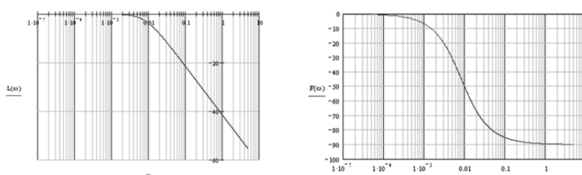
Рис. 3. Логарифмическая амплитудно-частотная характеристика и фазо-частотная характеристика
