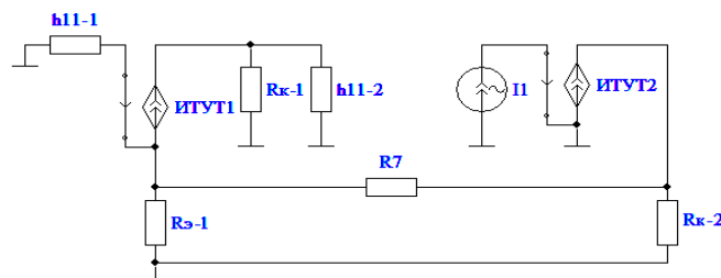
Рис. 5. Разрыв петли ОС в активной части цепи с независимым источником тока
