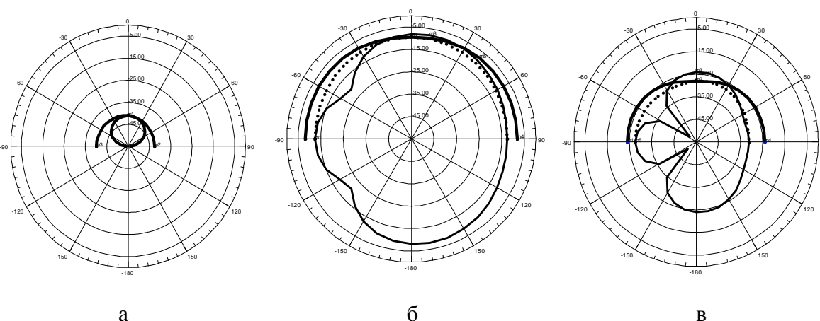
Рис. 2. Диаграмма направленности копланарного волновода (а), прямоугольного излучателя (б), антенной системы с копланарным волноводом (в)
