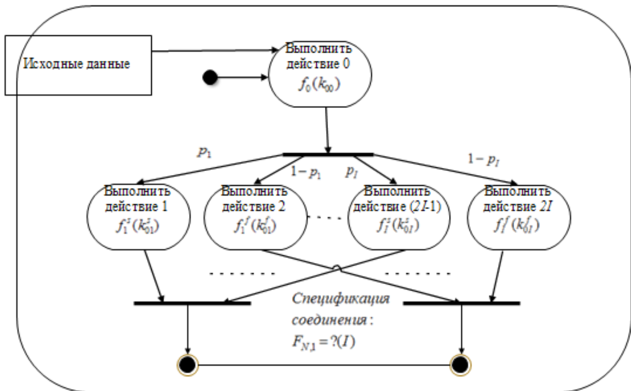
Рисунок. Диаграмма деятельности программного интеллектуального агента по достижению целей в информационной сети при априорно неопределённом механизме синхронизации распараллеленных действий
