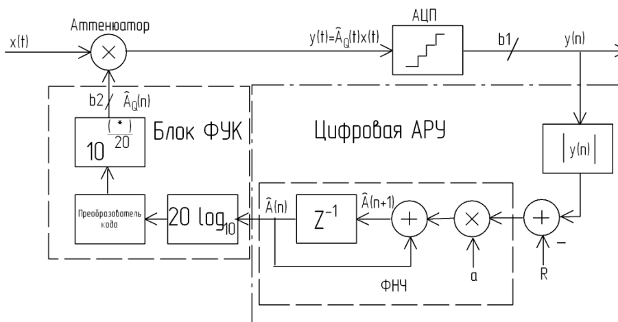
Рис. 1. Структурная схема модели ЦАРУ и тракта ПЧ ЦРПРУ
