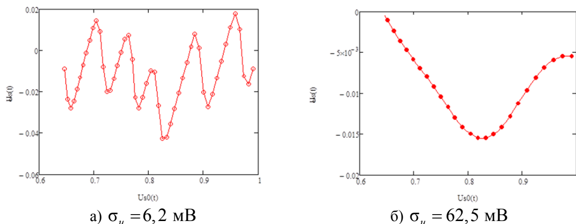
Рис. 2. Систематическая погрешность при нелинейном аналого-цифровом преобразовании
