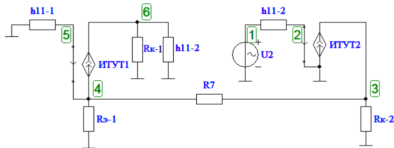
Рис. 4. Разрыв петли ОС в активной части цепи с независимым источником ЭДС
