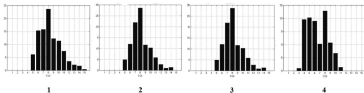
Рис. 5. Карты распределения CQI по площади соты
