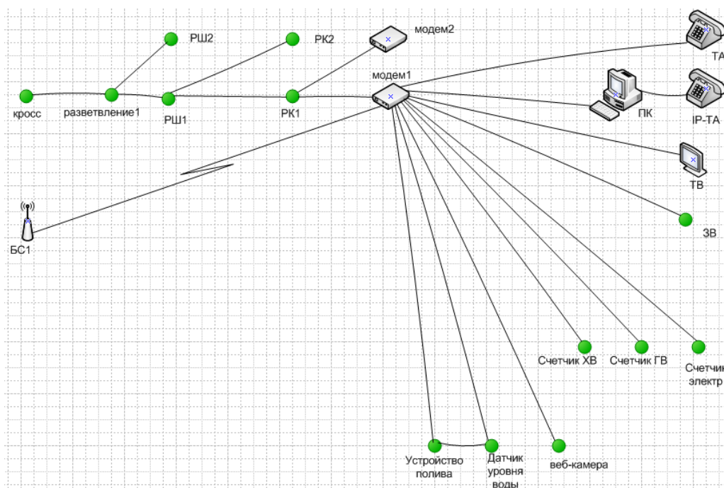
Рис. 1. Схема первичной сети G0
