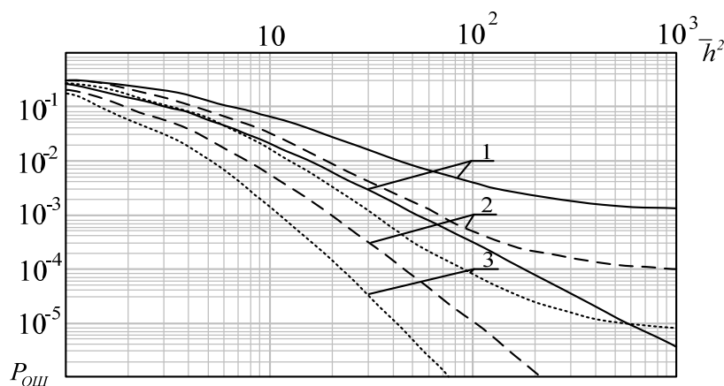
Рис. 2. Зависимости P_{\text{ош}} = \psi(\bar{h}^2) для НК схемы НК квадратичного сложения сигналов пришедших по: 1 – двум, 2 – трем и 3 – четырем дискретным лучам при отсутствии и наличии одновременно боковых пиков АКФ и ВКФ, равных значению ( \rho_{11\max} = 0,3 \rho_{10\max} = 0,3 )
