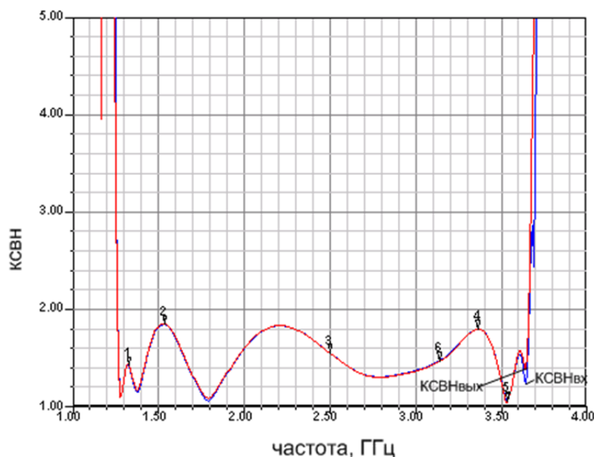
Рис. 4. КСВН входа/выхода фильтра после оптимизации
