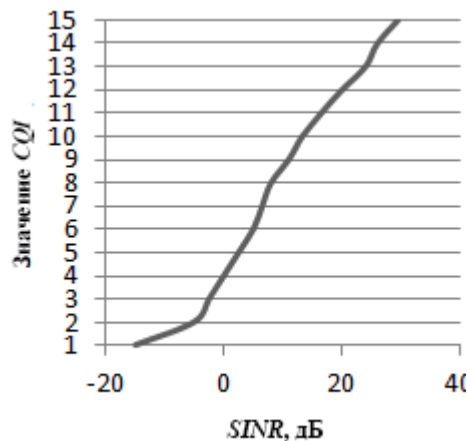
Рис. 4. Зависимость параметра CQI от величины SINR
