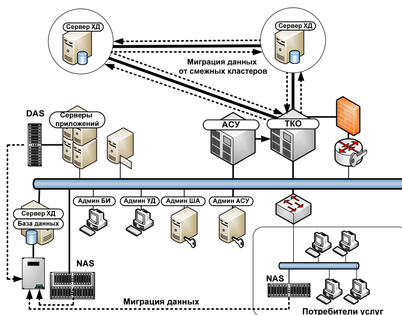
Рис. 1. Архитектура кластера системы хранения данных (вариант)
