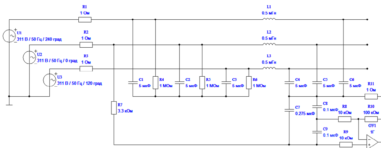
Рис. 3. Компьютерная модель ФРП с компенсацией тока утечки
