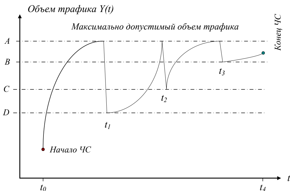
Рисунок. Алгоритм ограничения трафика в ЧС
