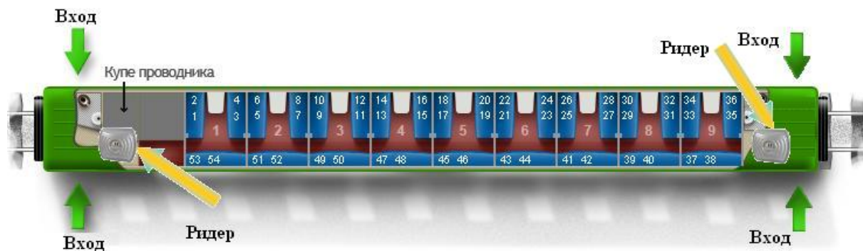
Рис. 2. Схема размещения ридеров
