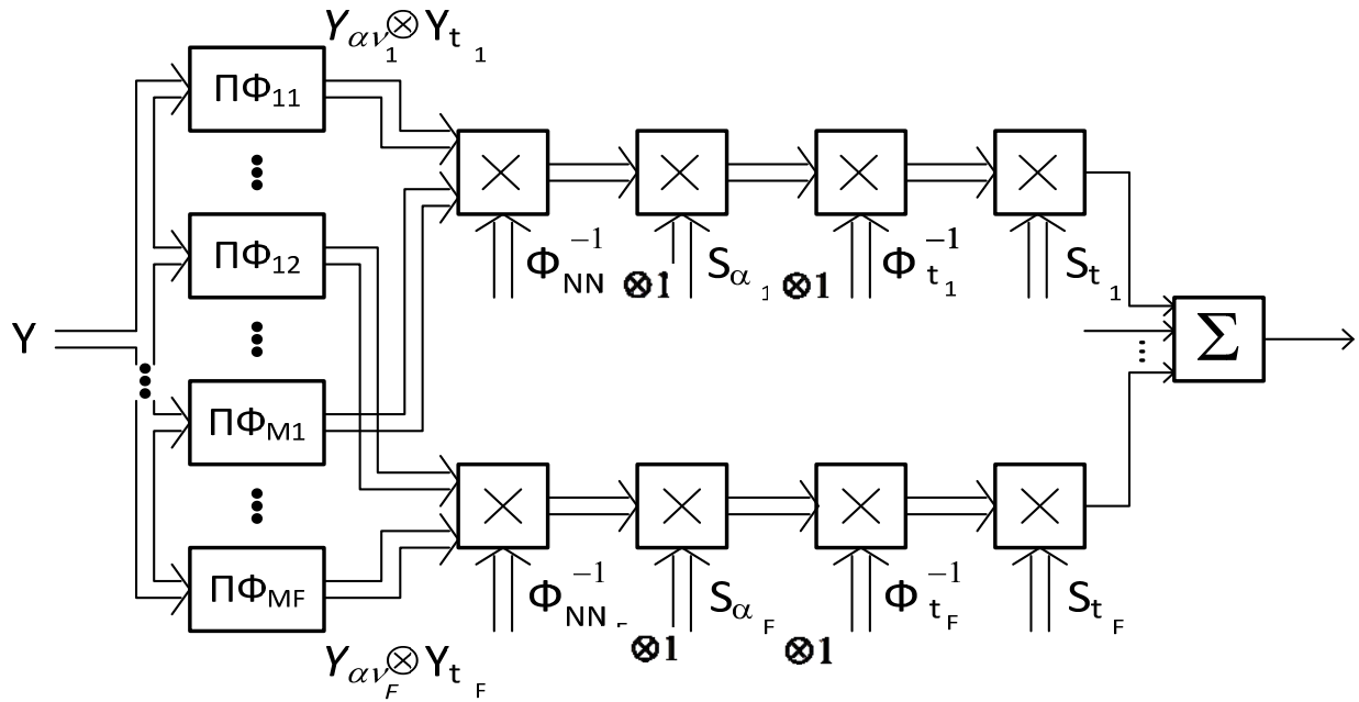
Рисунок. Структурная схема, реализующая факторизуемую пространственно-временную обработку
