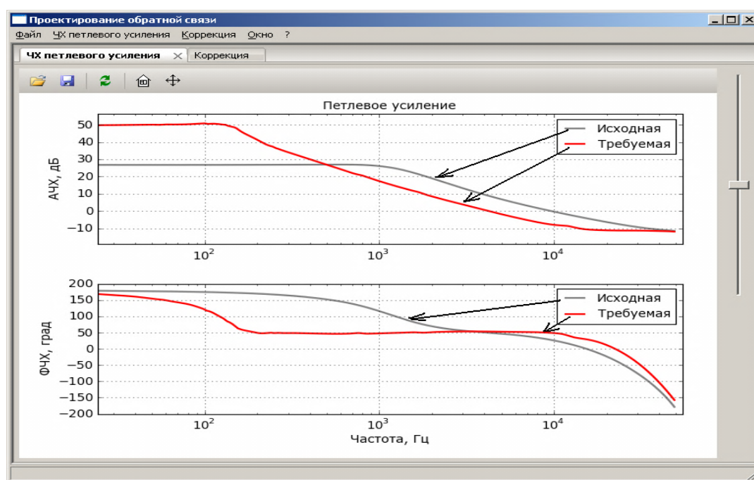
Рис. 4. Проектирование частотных характеристик петлевого усиления, оптимальных в смысле Боде
