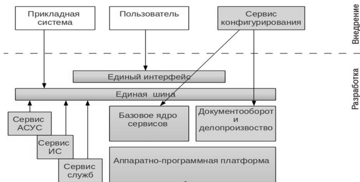
Рисунок. Общий вид инвариантной ИТКС
