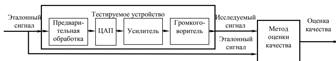
Рисунок. Схема исследовательской установки
