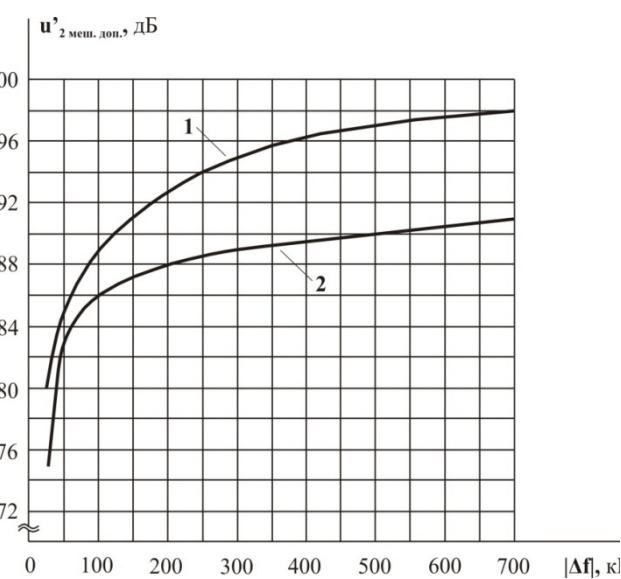
Рис. 2. Зависимости допустимого уровня мешающего сигнала по блокированию от частотного разнеса при полезном сигнале 1 мкВ и при избирательности по соседнему каналу 80 и 75 дБ
