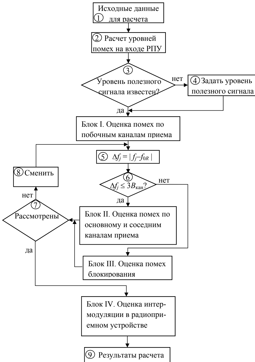
Рисунок. Структурная схема анализа ЭМС по результатам радиоконтроля
