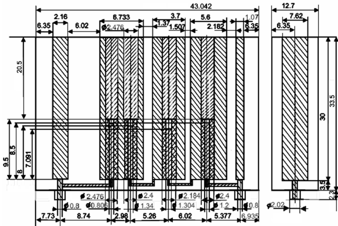
Рис. 2. Конструкция фильтра с геометрическими размерами
