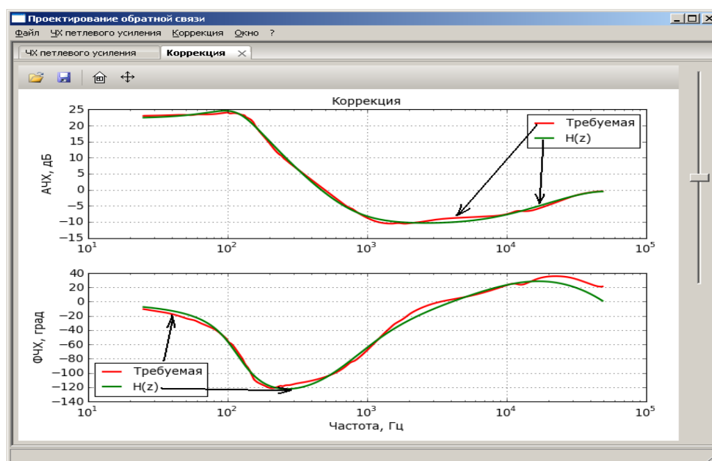
Рис. 5. Требуемые и синтезированные частотные характеристики цифрового корректирующего звена
