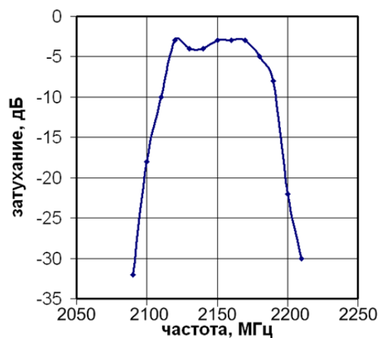
Рис. 2. Экспериментальная характеристика затухания лабораторного макета ступенчатого ЭФ с подключением двух горизонтальных разъемов до оптимизации
