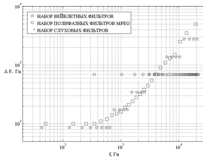
Рис. 3. Наборы различных полосовых фильтров [1]
