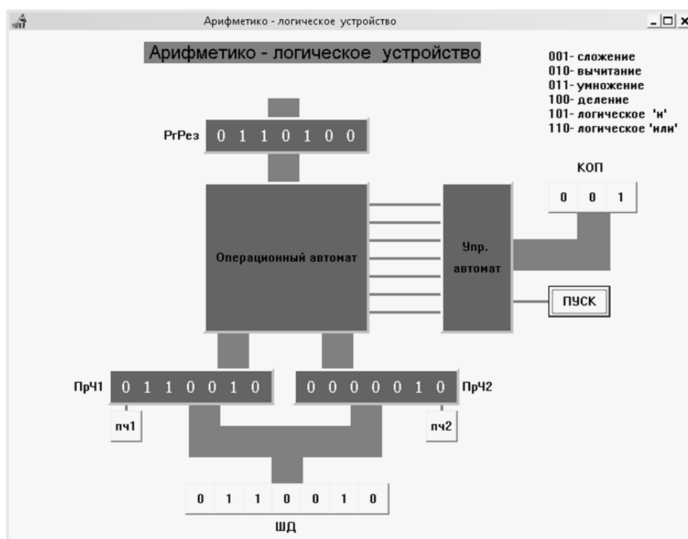
Рис. 1. Управляемая модель арифметико-логического устройства
