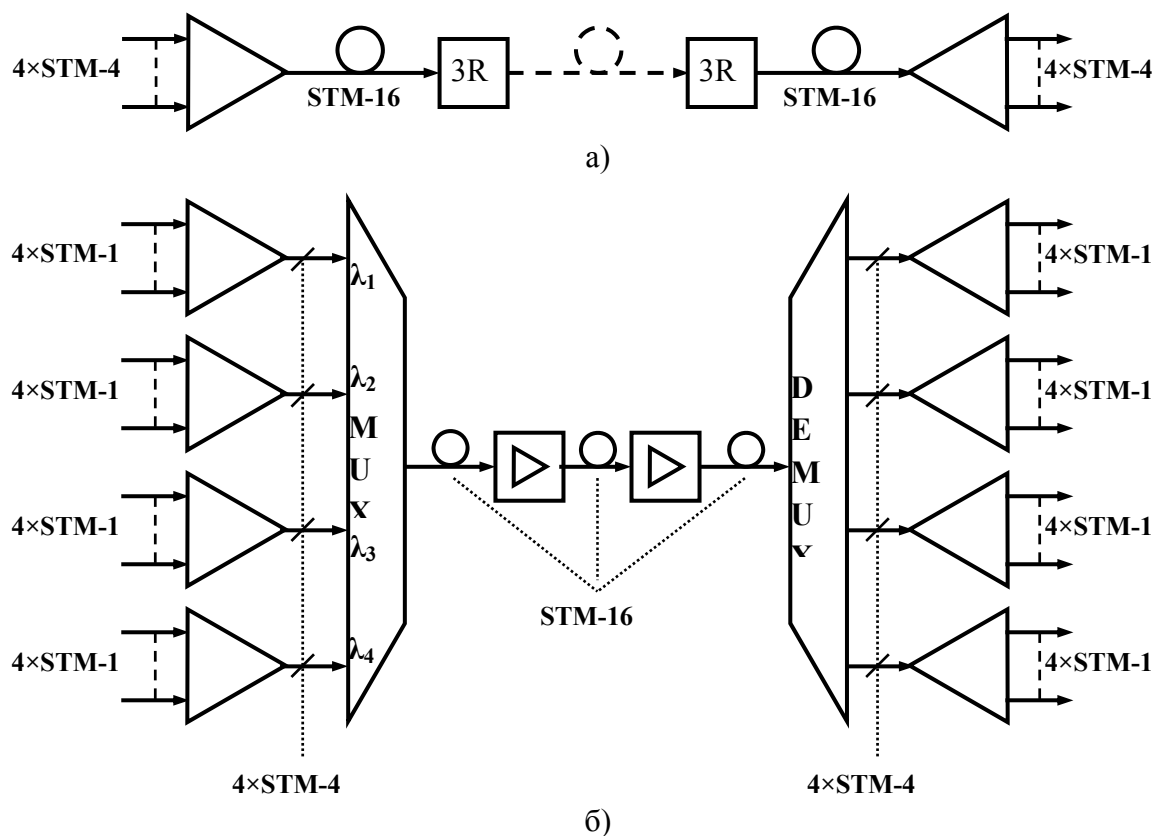
Рис. 2. К обсуждению принципов разделения сигналов: а) TDM, б) WDM
