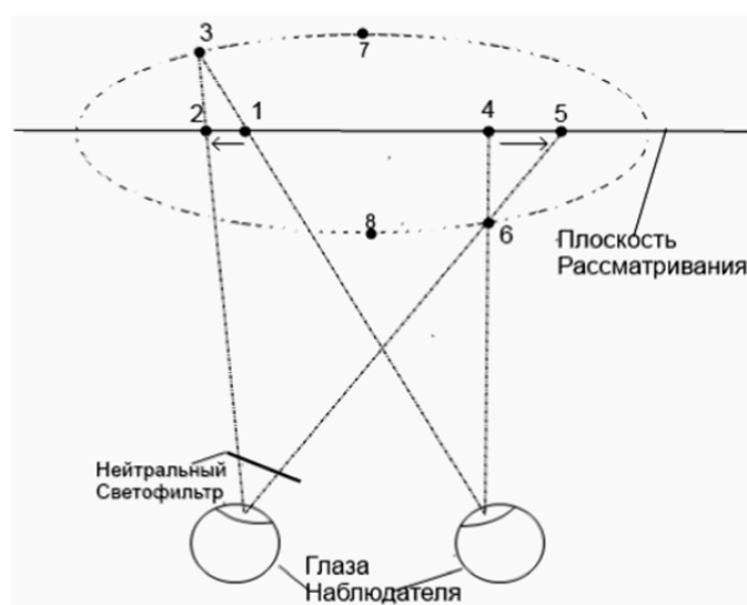
Рис. 3. Классическая схема опыта с маятником для демонстрации эффекта Пульфриха
