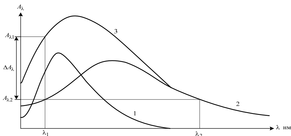
Рис. 2. Спектры поглощения к примеру 2:
