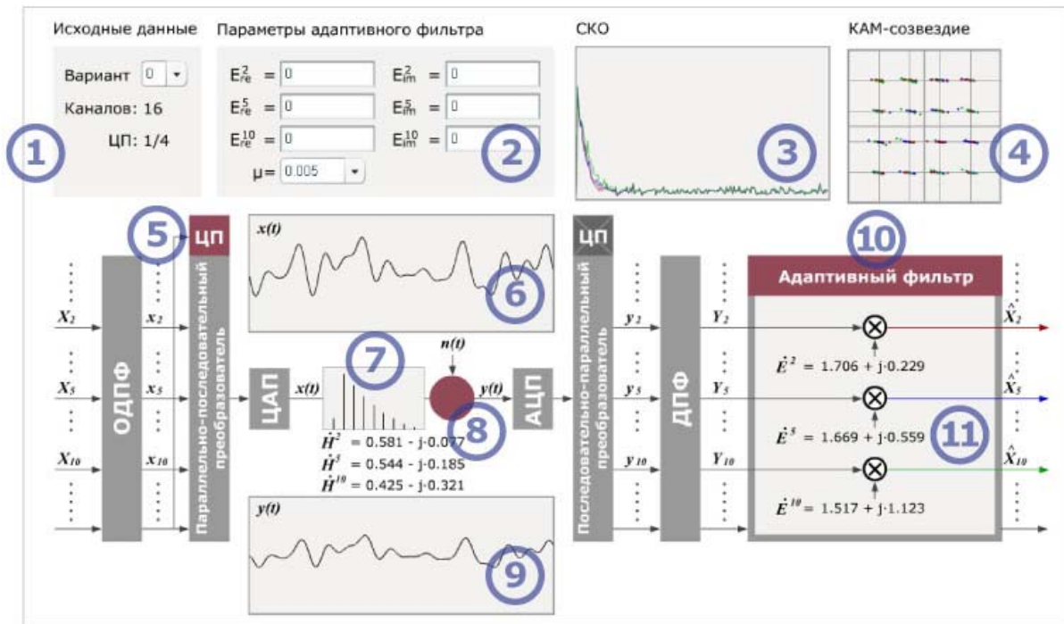
Рис. 1. Рабочий экран программы лабораторной работы
