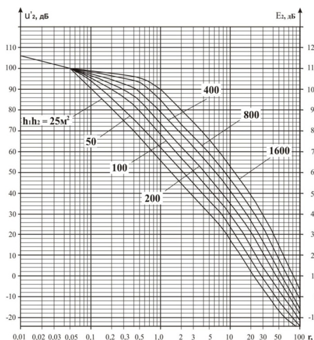
Рис. 1. Базовые кривые распространения для расчета кривых на станциях
