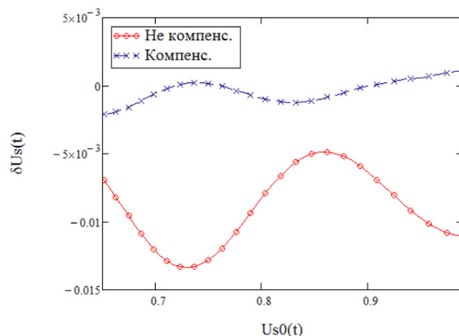
Рис. 3. Систематическая погрешность с компенсацией нелинейности шкалы АЦП
