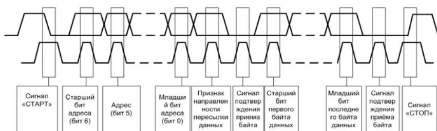
Рис. 2. Временная диаграмма обмена данными по интерфейсу I^2C
