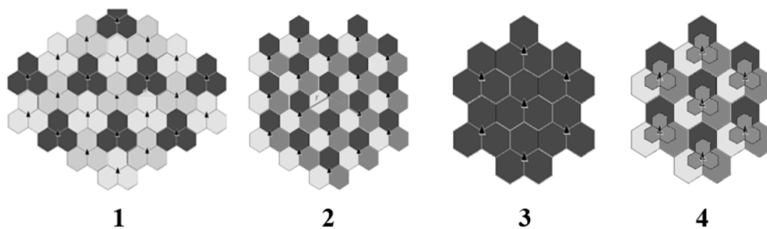
Рис. 1. Варианты распределения частотного ресурса между eNodeB
