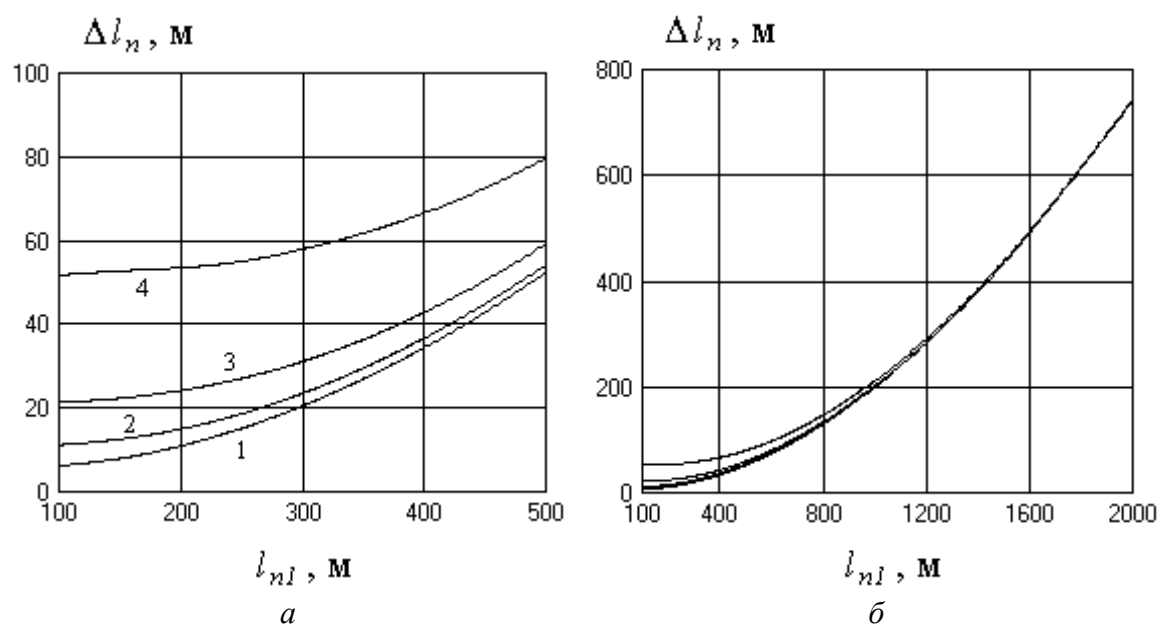
Рис. 3. Зависимости разрешающей способности от расстояния до первой неоднородности в кабеле ТПП-0.4 при различных длительностях зондирующего импульса: 1 – 50 нс, 2 – 100 нс, 3 – 200 нс, 4 – 500 нс
