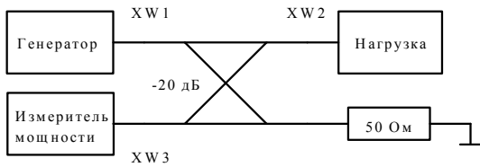
Рис. 2. Структурная схема контрольного тракта ФАР. Отраженный от нагрузки сигнал не должен попадать в измеритель мощности
