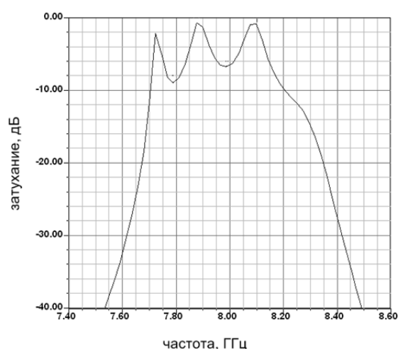
Рис. 2. Характеристика затухания гребенчатого фильтра 5-го порядка с цилиндрическими резонаторами по результатам моделирования до оптимизации
