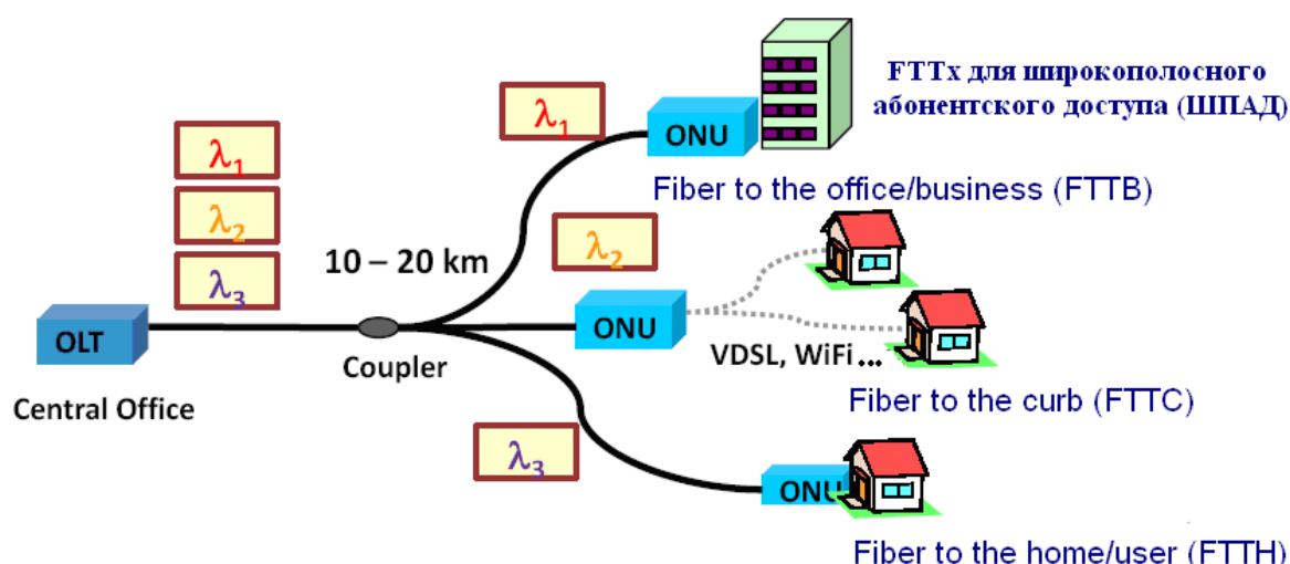
Рис. 2. Технология WDM-PON
