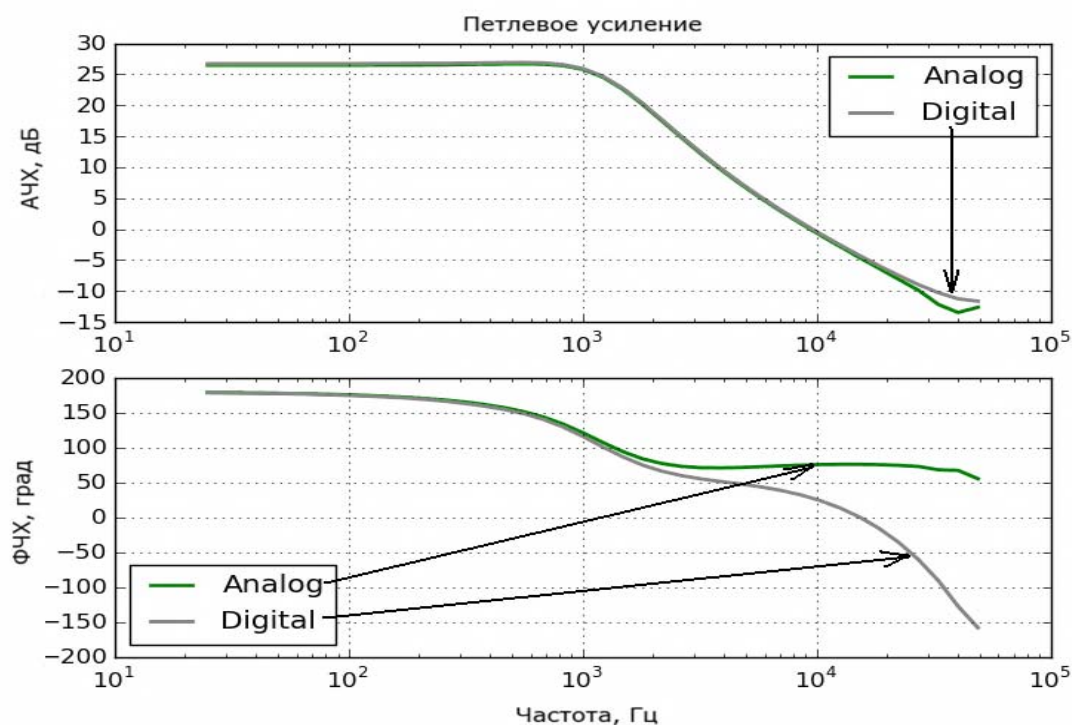
Рис. 3. Частотные характеристики петлевого усиления аналоговой и цифровой цепей ООС (без коррекции)
