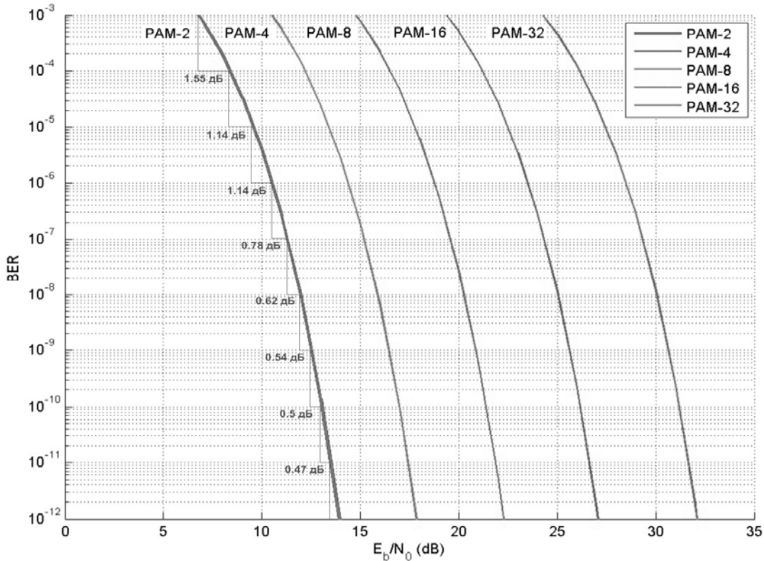
Рис. 1. Зависимость SNR от BER
