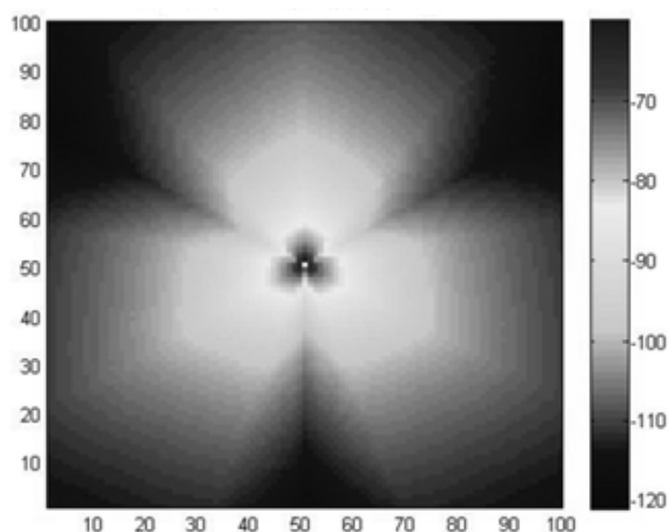
Рис. 3. Диаграмма уровней затухания сигнала (в децибелах)
