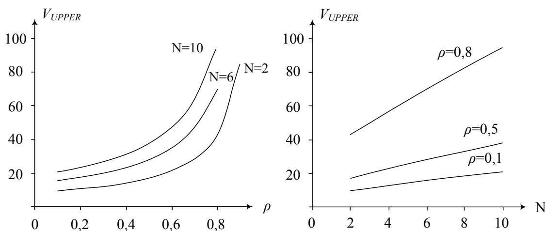
Рисунок. Зависимость квантиля V_{UPPER} от загрузки и числа фаз
