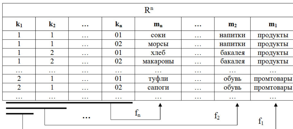
Рис. 1. 1NF отношение R^n с рекурсивными потенциальными ключами и цепочно вложенными функциональными зависимостями
