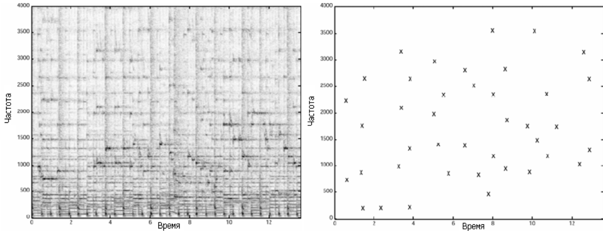
Рис. 3. Спектрограмма сигнала (слева) и «карта созвездий» полученная в результате прореживания (справа)
