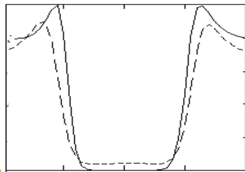
Рис. 4. Сплошная линия – амплитудно-частотная характеристика идеального эллиптического полосового фильтра, пунктирная – расчетная амплитудно-частотная характеристика фильтра на линиях с учетом дисперсии и потерь. Ширина полосы пропускания 4 %
