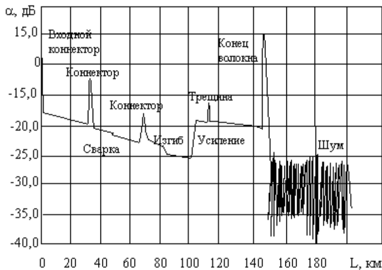
Рис. 4. Рефлектограмма ОВ
