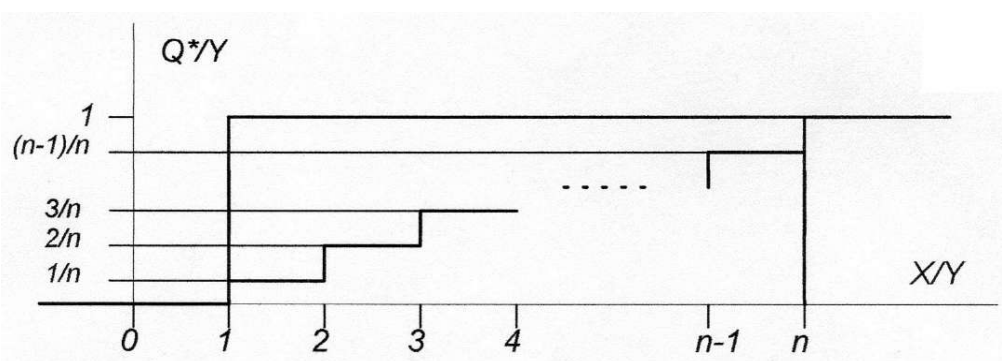
Рисунок. Зависимости относительной гарантируемой реализованной нагрузки Q^*/Y от соотношения суммарной пропускной способности транспортной сети X и суммарной нагрузки Y
