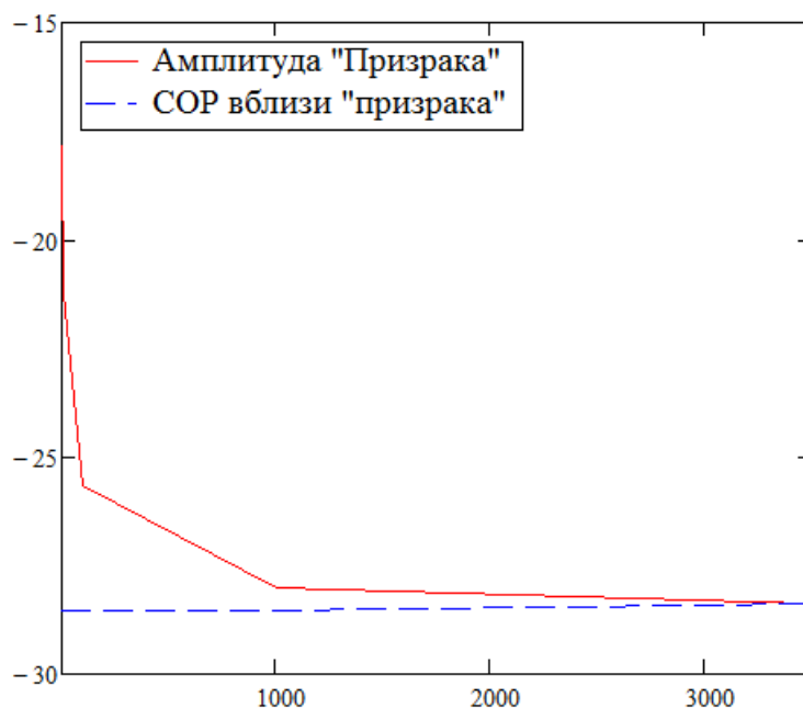
Рис. 5. Зависимость амплитуды «призрака» от числа накоплений
