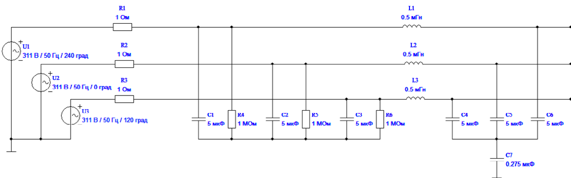
Рис. 1. Компьютерная модель ФРП для 3-х фазной сети
