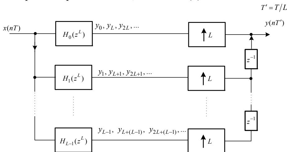
Рис. 2. Полифазная структура системы однократной интерполяции
