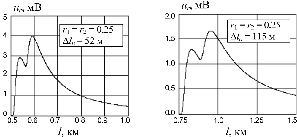
Рис. 1. Фрагменты рефлектограмм кабельных цепей. Расчет произведен для кабеля ТПП-0.4 при амплитуде зондирующего импульса 1 В, длительности 50 нс и расстояниях до первой неоднородности l_{n1} : 0.5 км (слева) и 0.75 км (справа)
