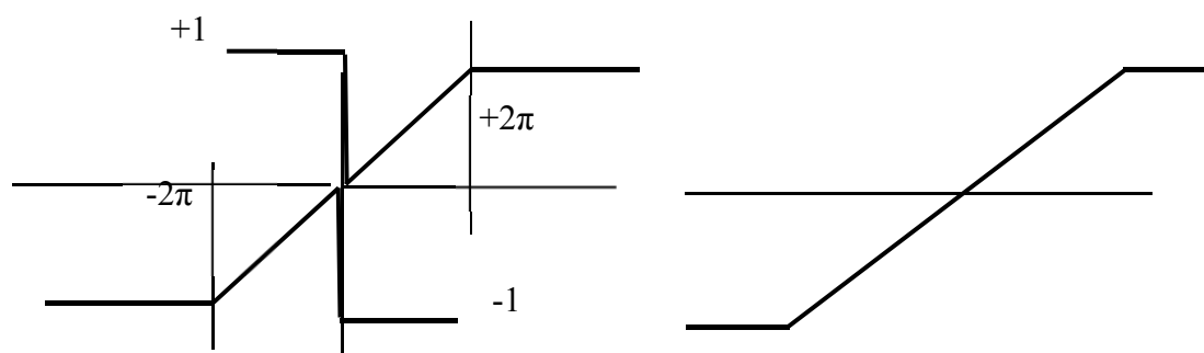
Рис. 1. «Сшивание» характеристики ЧФД
