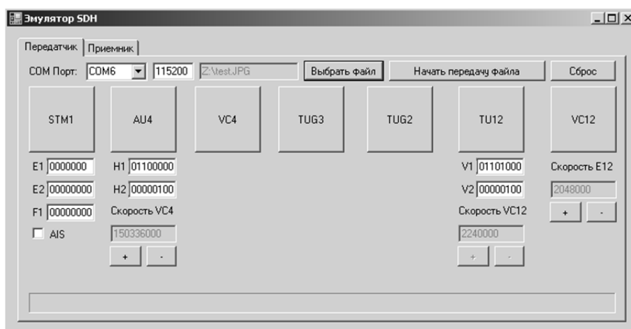
Рис. 1. Интерфейс программы. Передатчик
