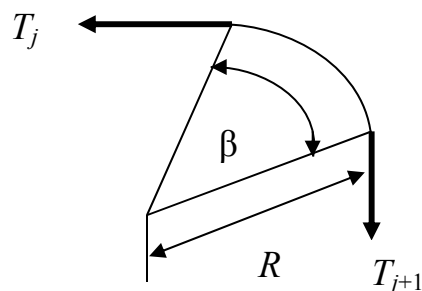
Рис. 2. Горизонтальный изгиб кабеля при прокладке
