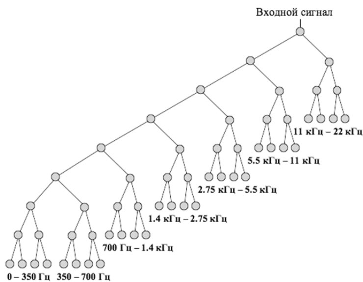
Рис. 2. Вариант дерева вейвлетной декомпозиции [1]
