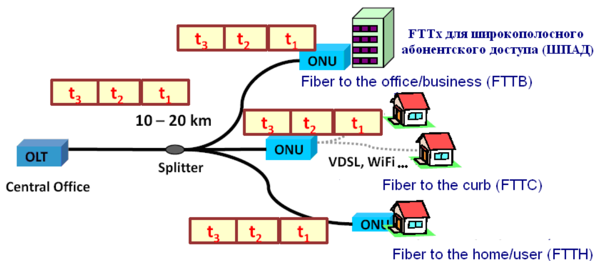
Рис. 1. Технология TDM-PON
