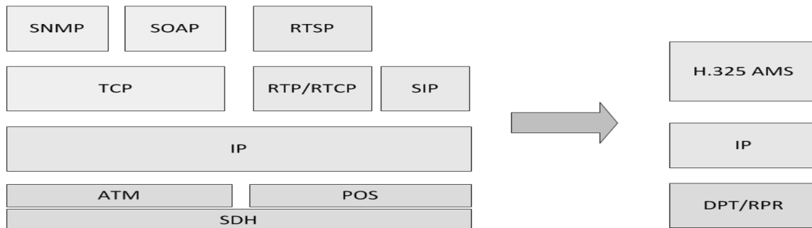
Рис. 5. Преобразование стека протоколов с использованием H.325 и DPT/RPR
