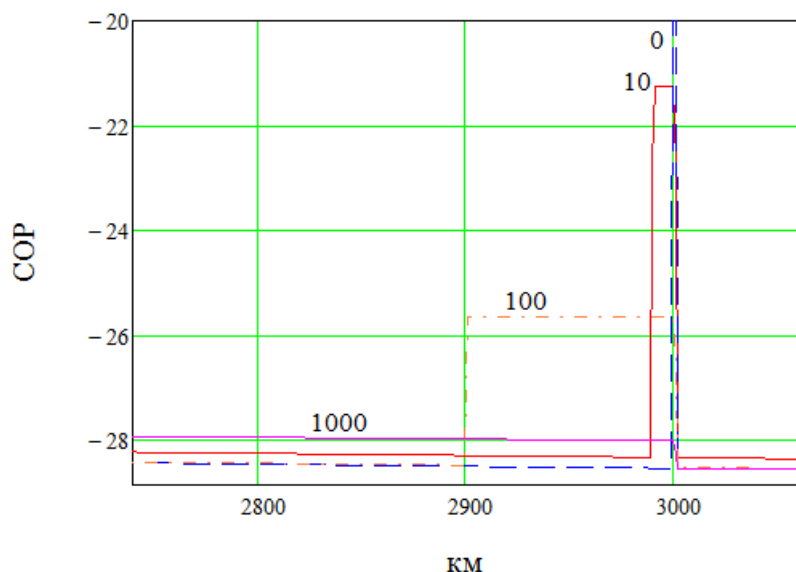
Рис. 4. Изменение амплитуды «призрака» при различном числе накопления
