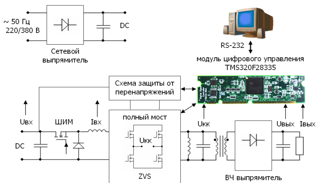
Рис. 1. Пример схемы DC-DC преобразователя на основе резонансного инвертора тока
