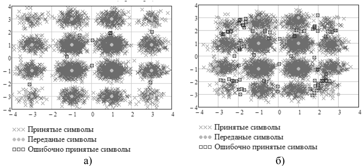
Рис. 2. Диаграмма рассеяния для N=4 при c\backslashш = 15 дБ
