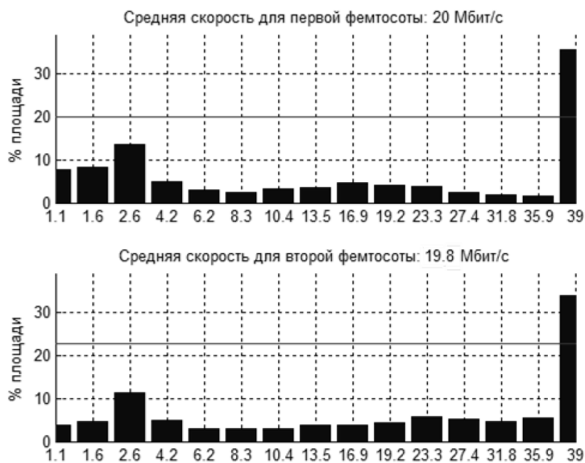
Рис. 7. Распределение скоростей доступа вниз (сценарий 4)
