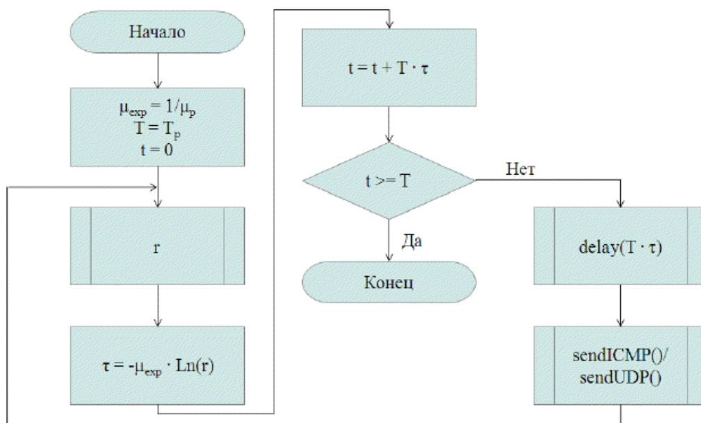
Рисунок. Алгоритм основной функции генерации пакетов по заданному распределению
