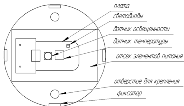
Рис. 1. Комбинированный датчик
