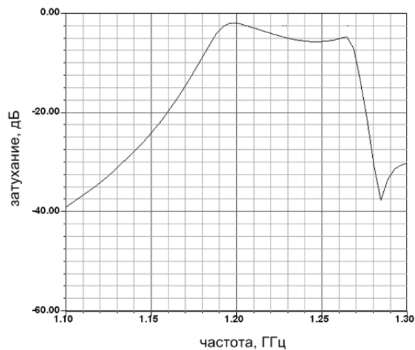
Рис. 2. Характеристика затухания микрополоскового фильтра 6-го порядка на встречных стержнях по результатам моделирования до оптимизации
