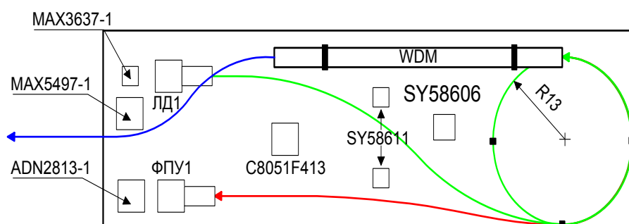
Рис. 3. Компановка платы ОУТ (Второй ОУТ расположен на другой поверхности платы, размер общей платы 100x30 мм)
