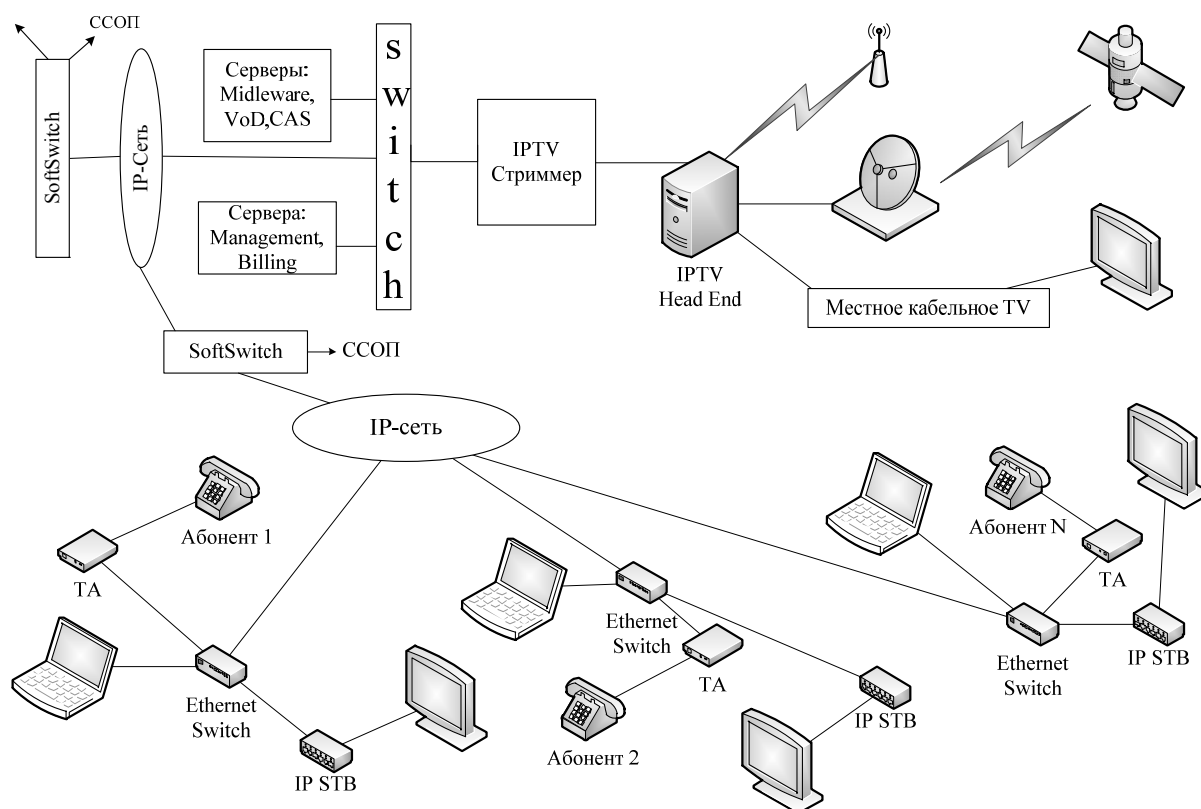
Рисунок. Базовая структура системы IPTV
