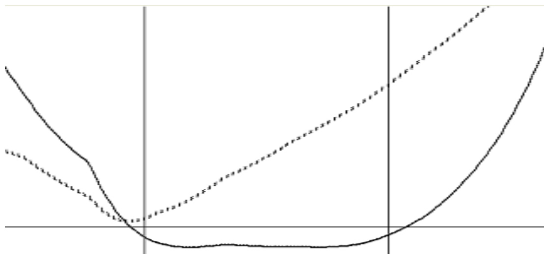
Рис. 3. Прерывистая линия – зависимость КСВ от частоты антенны, сплошная – расчетная зависимость КСВ от частоты при согласовании антенны согласующим устройством из трех последовательно включенных отрезков компланарного волновода, с меняющимся по экспоненциальному закону волновым сопротивлением. В полосе частот (2,1–2,45 ГГц) КСВ меньше 1,5 (горизонтальная линия).
