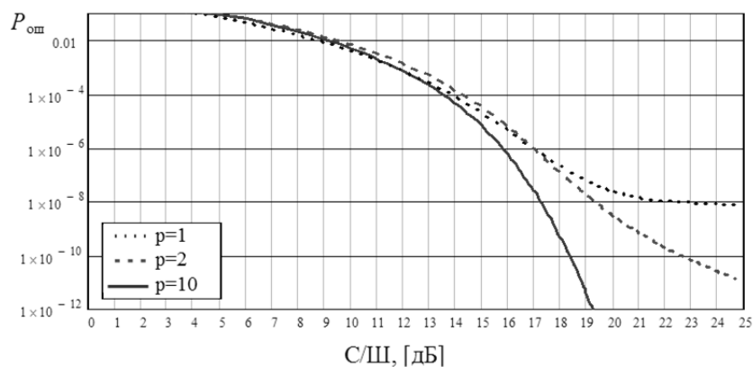
Рис. 3. Рабочая характеристика канального селектора
