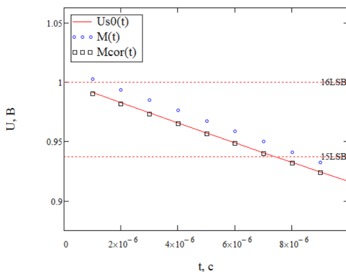
Рис. 4. Исходная рефлектограмма и результат её преобразования
