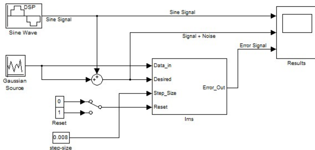
Рис. 1. Схема исследования эхо подавителя на Matlabe
