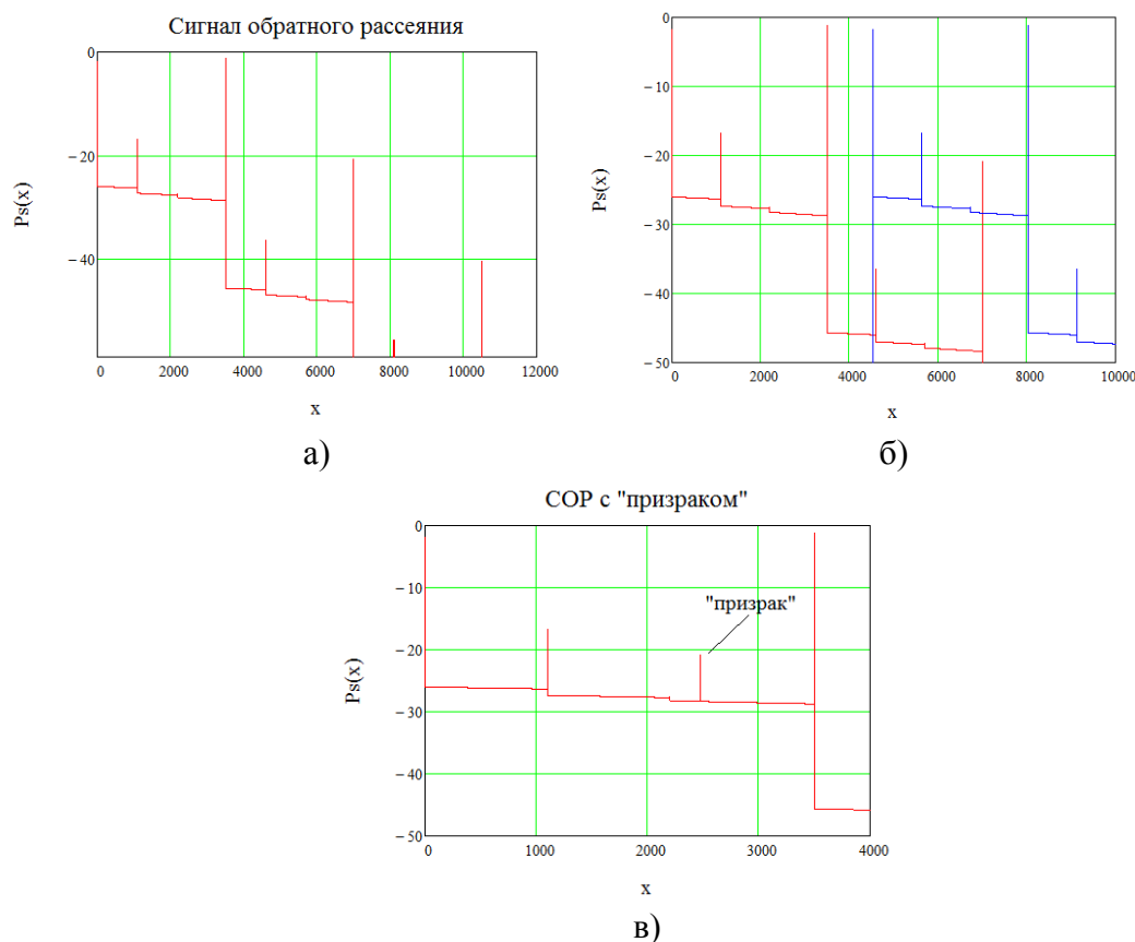
Рис. 3. Сигнал обратного рассеяния с «призраком»
