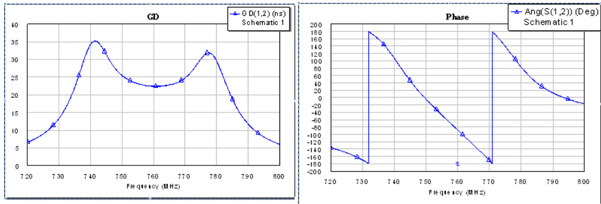
Рис. 7. Характеристика ГВЗ фильтра и ФЧХ фильтра
