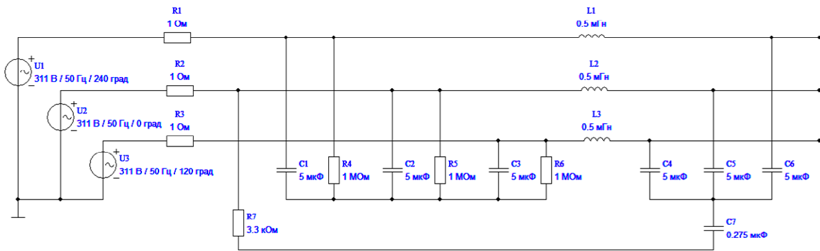
Рис. 2. Схема измерения тока утечки
