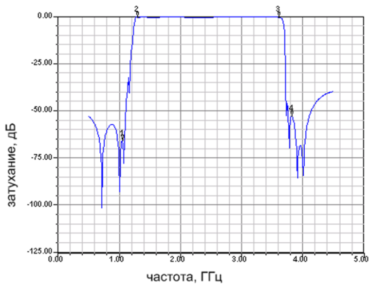
Рис. 3. Характеристика затухания фильтра после оптимизации
