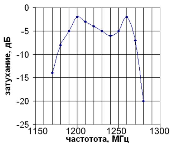
Рис. 3. Экспериментальная характеристика затухания макета микрополоскового фильтра 6-го порядка на встречных стержнях до оптимизации
