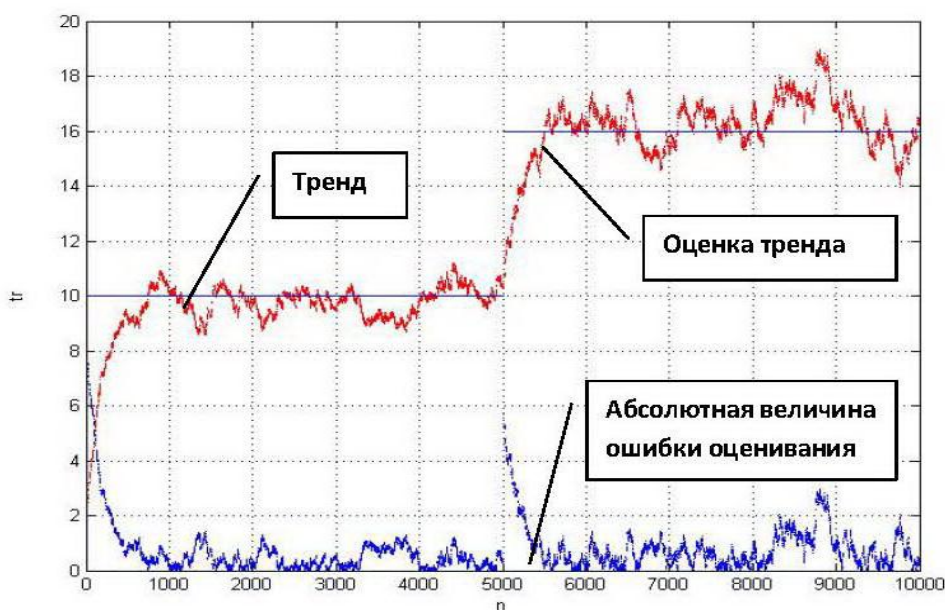
Рис. 1. Оценка ступенчатого тренда алгоритмом МСА
