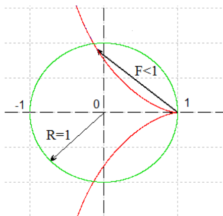
Рис. 5. Единичная окружность в увеличенном масштабе
