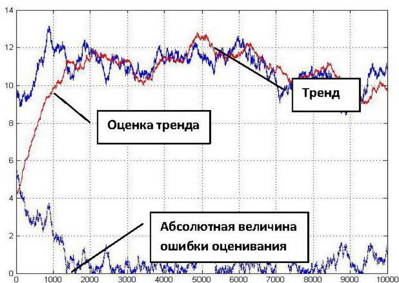
Рис. 2. Оценка случайного (процесс АРР первого порядка) тренда алгоритмом МСА
