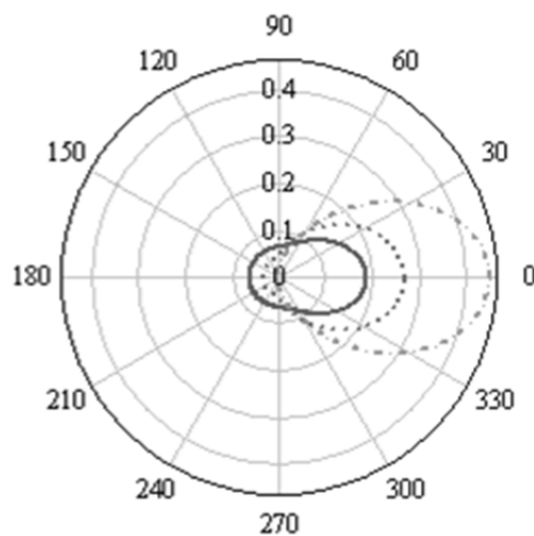
Рис. 2. Диаграмма нормированной индикатрисы рассеяния хиломикронов (сплошная – \rho_{ср} = 1 ; точечная – \rho_{ср} = 1,5 ; штрихпунктирная – \rho_{ср} = 2 )
