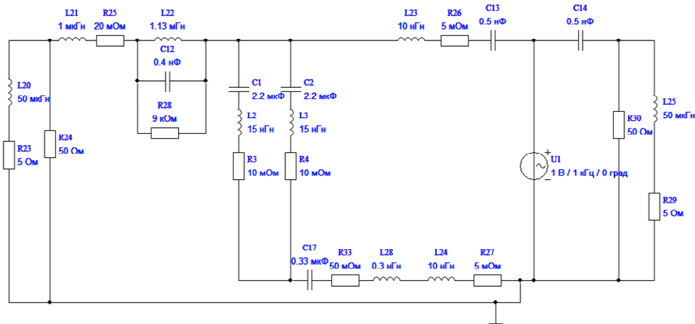
Рис. 7. Схема замещения ФРП для несимметричных помех
