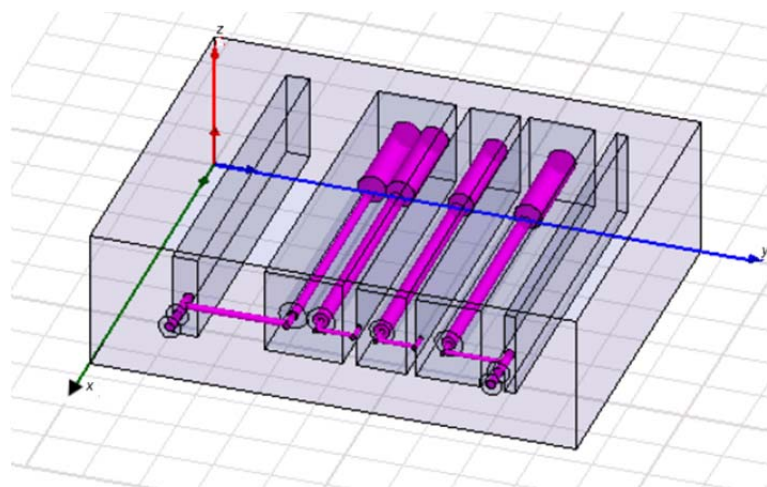
Рис. 1. 3D- модель фильтра
