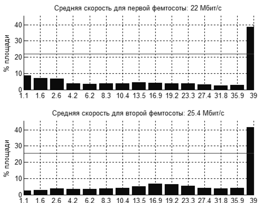
Рис. 5. Распределение скоростей доступа вниз (сценарий 3)
