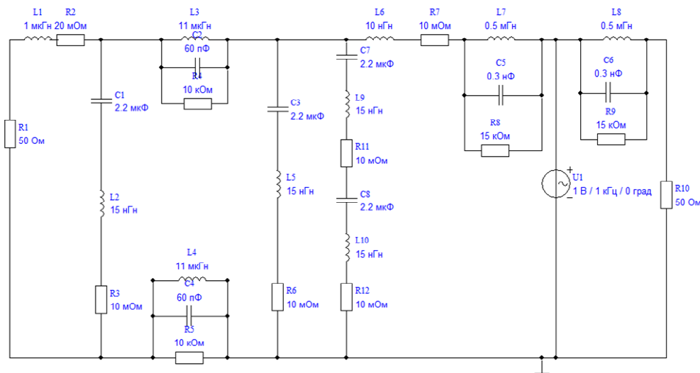
Рис. 8. Схема замещения ФРП для симметричных помех
