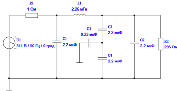
Рис. 6. Компьютерная модель ФРП
