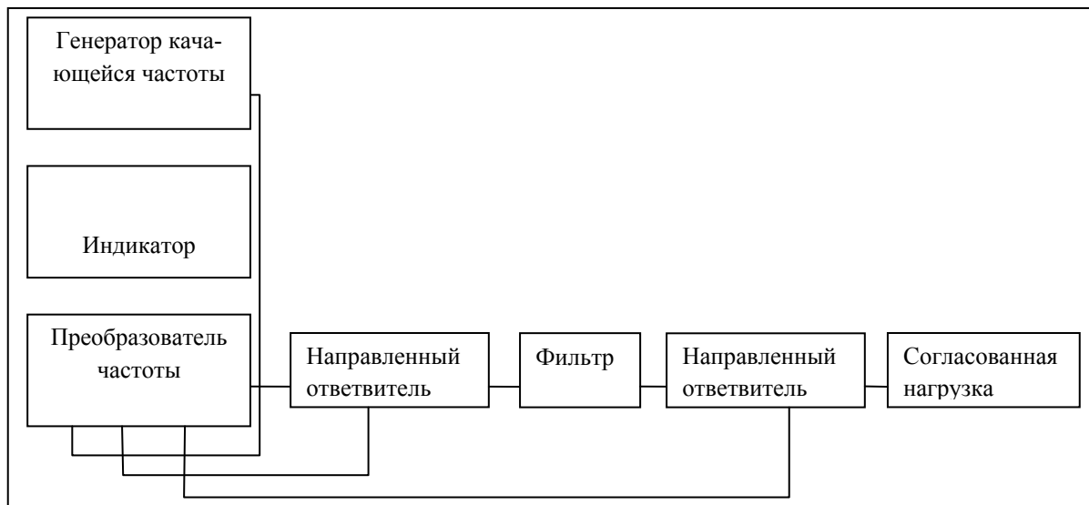
Рис. 2. Схема установки «Измеритель комплексных коэффициентов передачи Р4-11»
