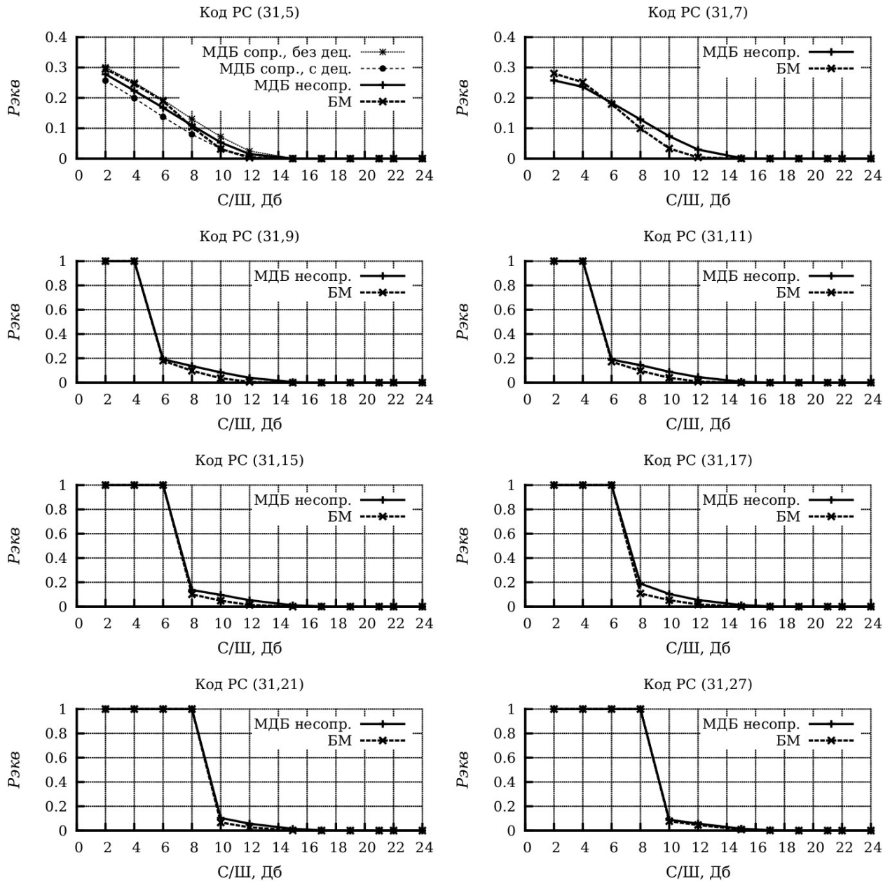
Рис. 2. Графики результатов оценки исправляющей способности алгоритма МДБ в сравнении с оценкой исправляющей способности алгебраического метода декодирования на основе алгоритма БМ
