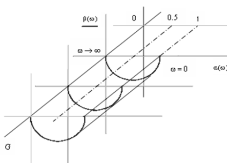
Рис. 4. Пространственный годограф пространственно-апериодического звена
