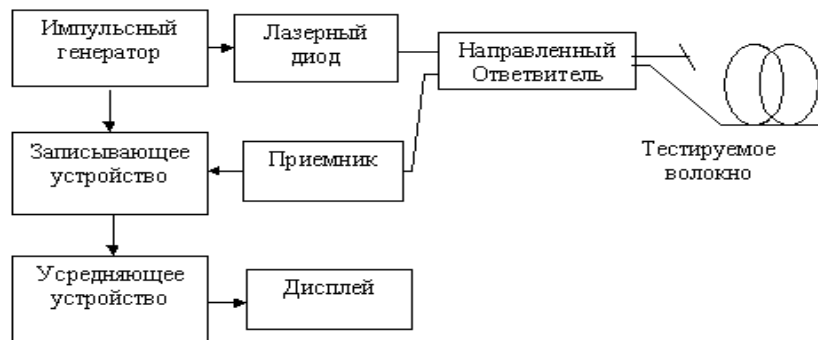
Рис. 3. Структурная схема оптического рефлектометра
