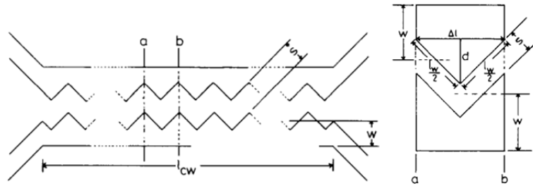
Рис. 3. Геометрические параметры зубчатых связанных линий
